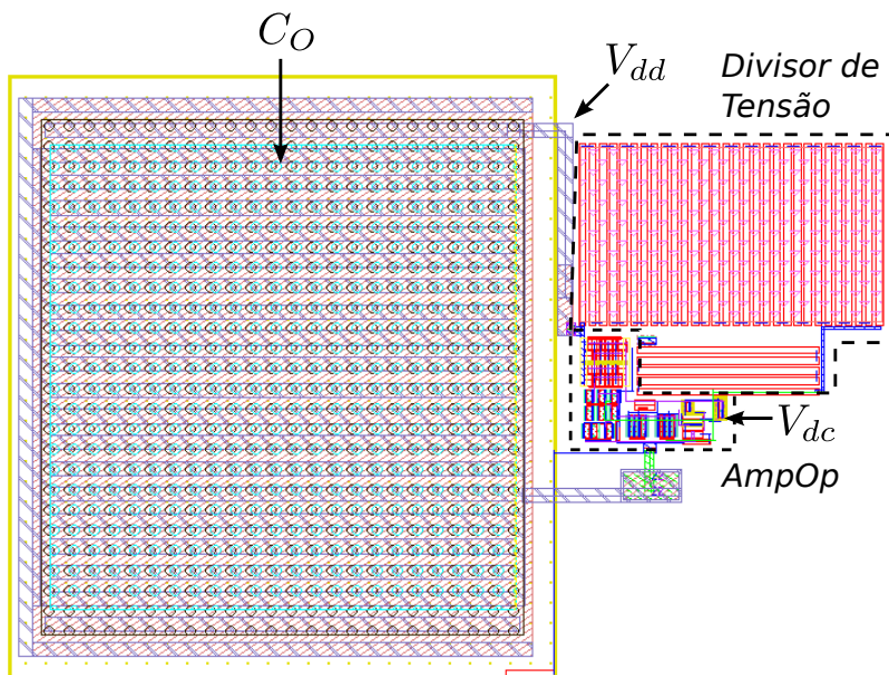
Figura 53: Layout do regulador de tensão (Área = 300 \mu\text{m} \times 137 \mu\text{m} )
