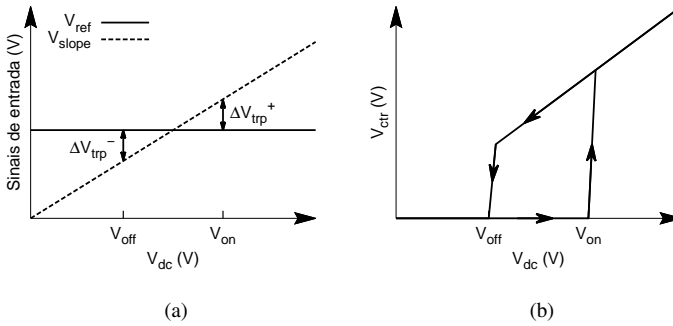
Figura 7: Sinais de (a) entrada e (b) saída ideais do seletor de modo de operação
