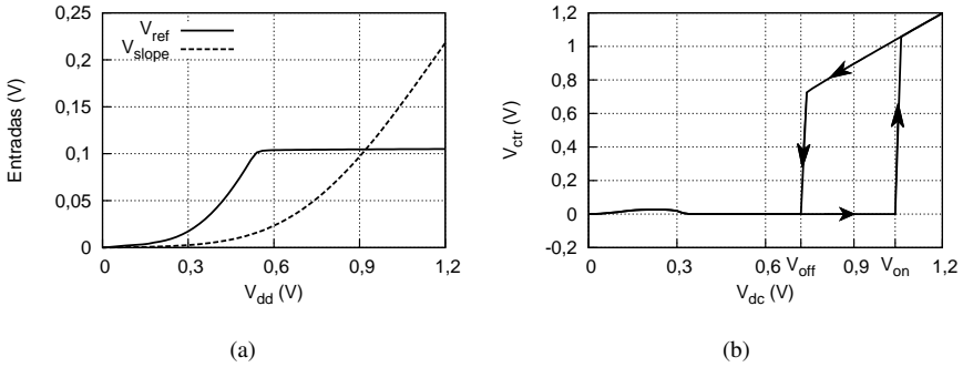
Figura 21: Sinais de (a) entradas e (b) saída do seletor de modo de operação com a alimentação variando do nível baixo para o alto e vice-versa (sentido indicado pelas setas)
