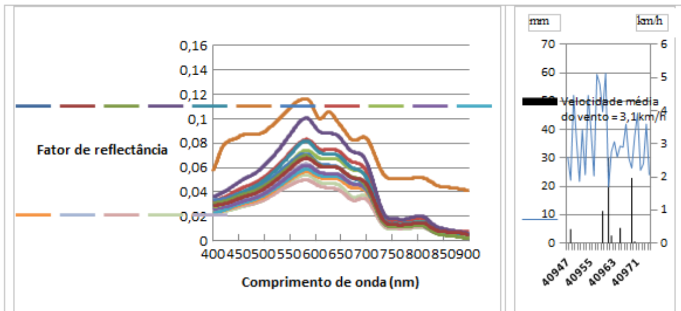
Figura 06 - Espectros de reflectância do Lago Guaíba (07/03/2012) e gráfico com os registros de chuva e velocidade do vento nos 30 dias que antecederam o trabalho de campo.
