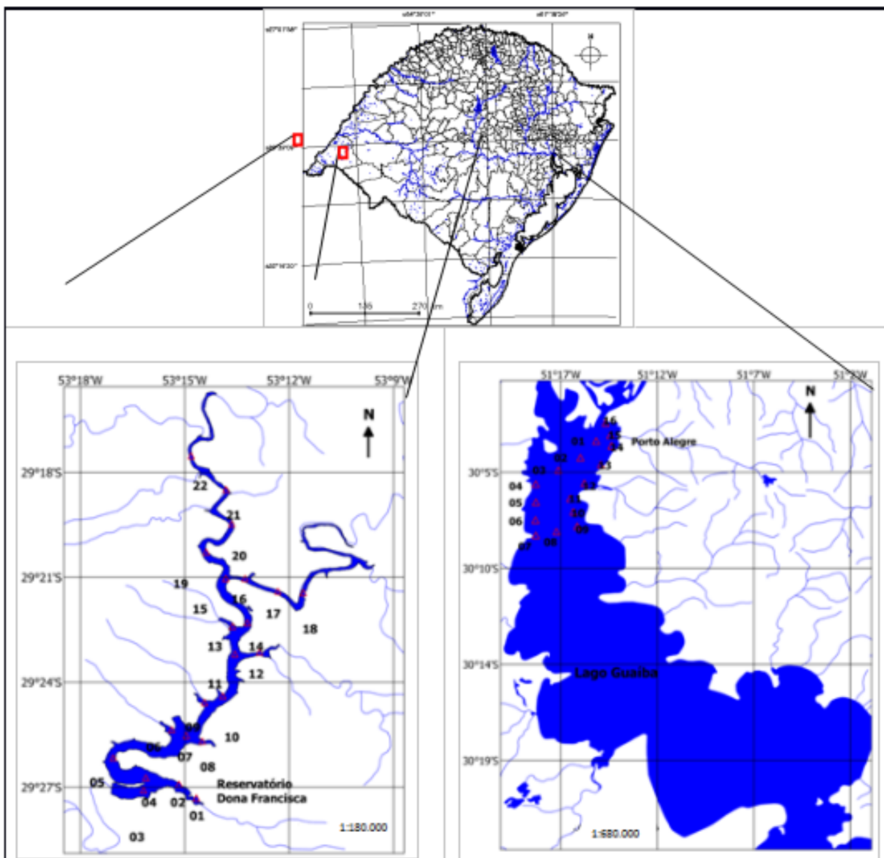
Figura 01 - Localização do reservatório Dona Francisca e do Lago Guaíba no estado do Rio Grande do Sul com destaque para a localização dos pontos amostrais.
