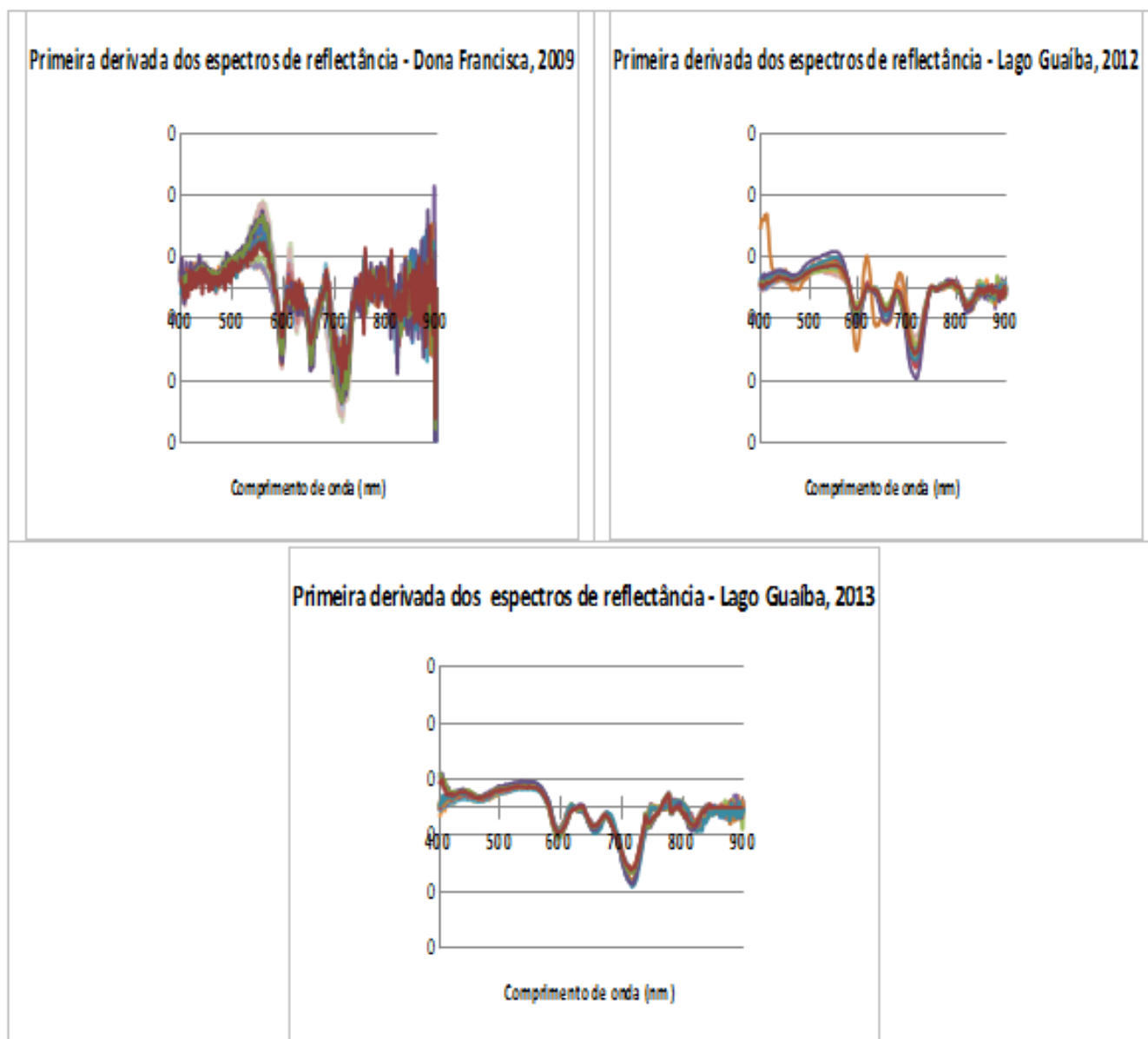
Figura 08 - Primeira derivada dos espectros de reflectância do reservatório Dona Francisca e do Lago Guaíba.
