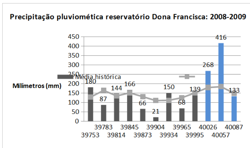
Figura 02 - Precipitação pluviométrica média mensal na bacia hidrográfica do reservatório Dona Francisca.
