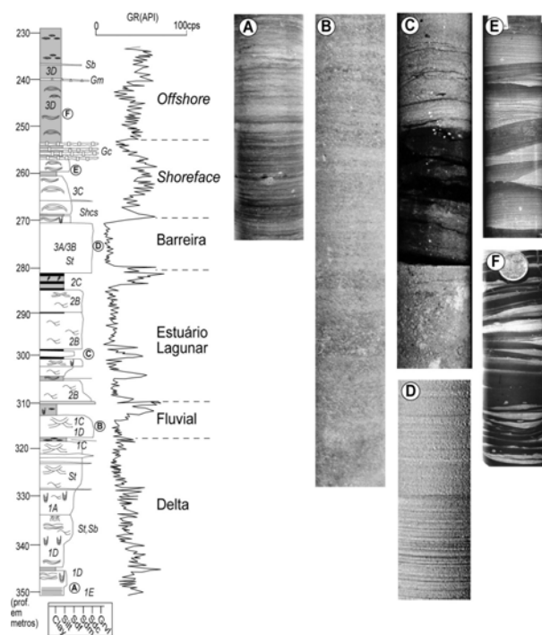
Figura 2 – Exemplo da sucessão estratigráfica em uma sondagem na área de estudo. O sistema de leque não ocorre, mas os principais sistemas deposicionais estão bem representados.
