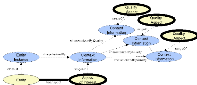
Figura 11: Representação de entidades de contexto e seus relacionamentos na ontologia CoOL Core [93]
