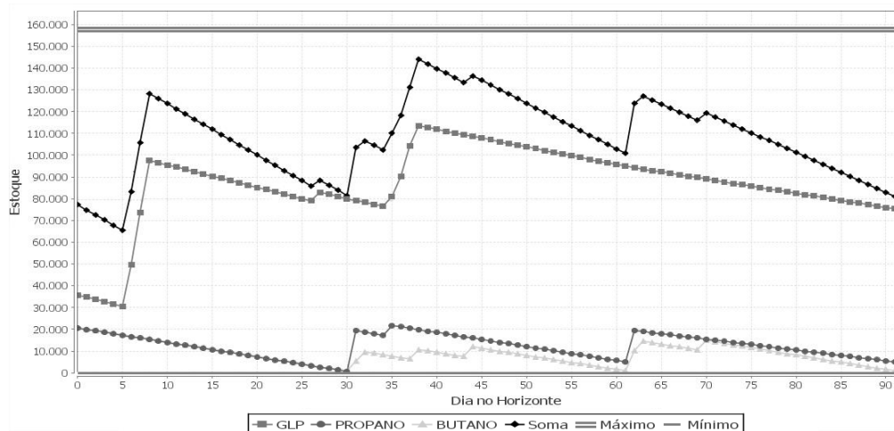
Figura 4. Curvas de estoque referentes ao agrupamento de GLP da região de São Paulo
