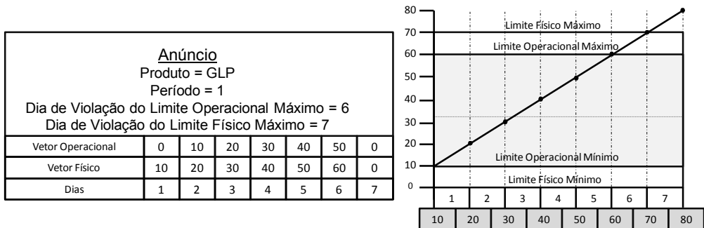
Figura 3. Representação do anúncio em relação à curva de estoque da tancagem.
