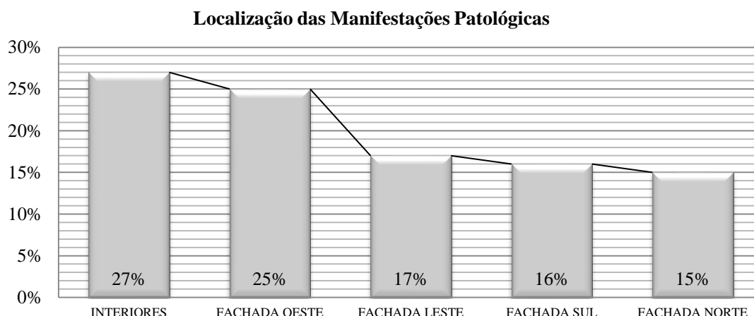
Figura 7 - Localização das manifestações patológicas ocorridas nas unidades habitacionais do conjunto construídas pela empresa A
