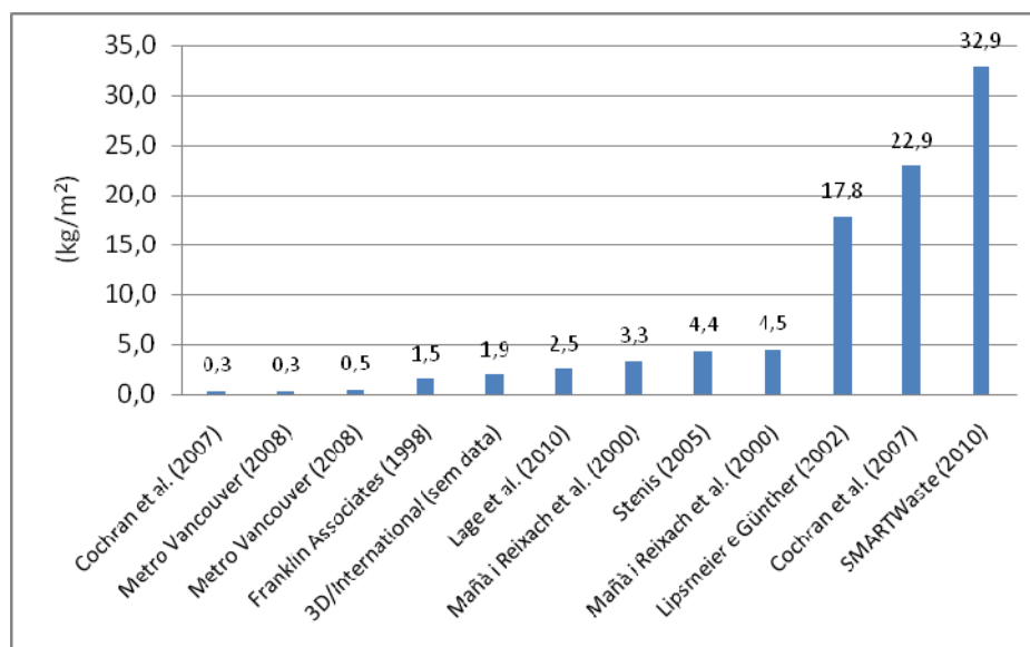
Figura 1 - Distribuição dos valores referentes ao código 17 01 01 (kg/m 2 )
