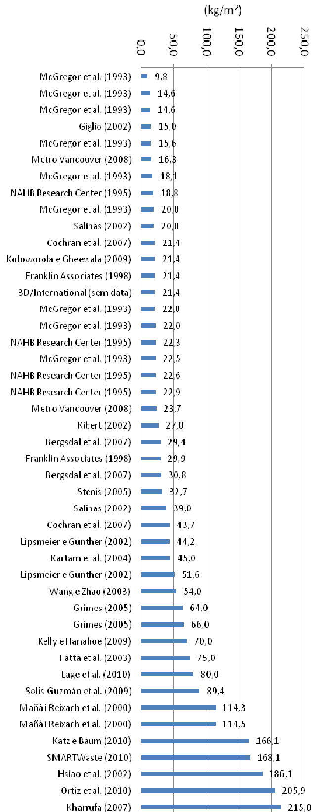
Figura 2 - Distribuição dos valores referentes à geração total de RCD (kg/m²)
