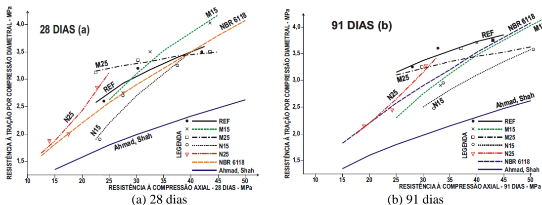
Figura 7 - Resistência à compressão diametral x compressão axial a 28 dias (a) e a 91 dias (b)
