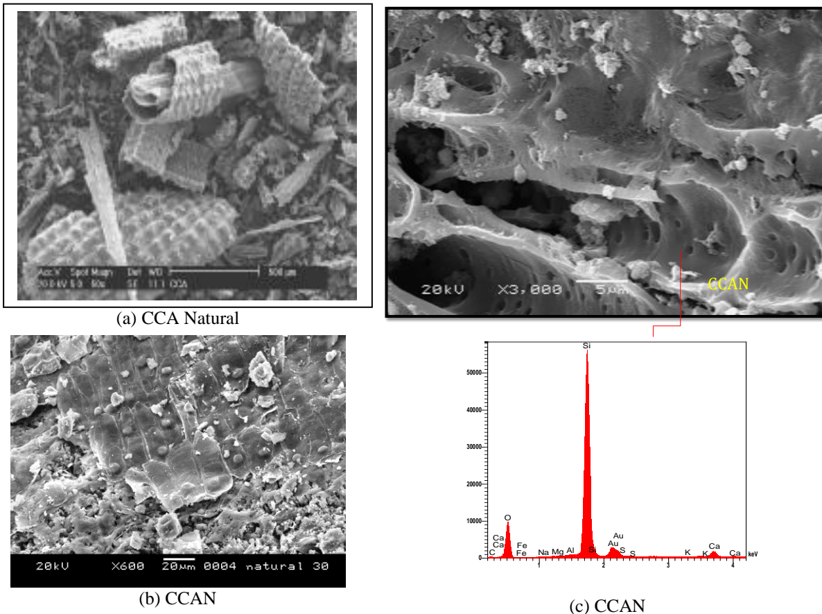
Figura 12 - (a) Epidermes internas e externas de CCA natural (b) e (c) Estruturas celulares remanescentes da lignina e celulose preenchidas com produtos de hidratação e/ou pozolânicos do traço CCAN
