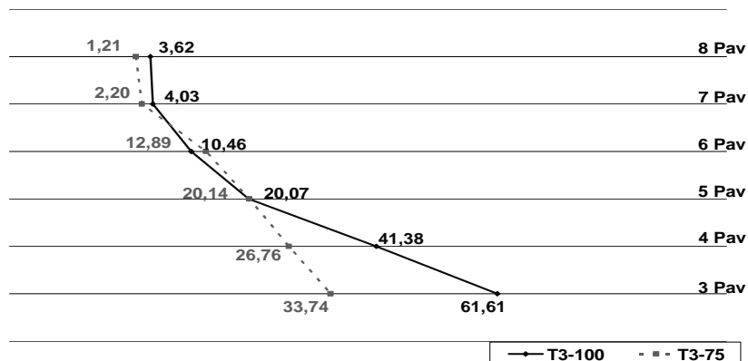
Figura 12 - Pressões positivas máximas, em mm.c.a., no tubo de queda para o arranjo de descarga Da e diâmetros de 100 mm e 75 mm para bacia sanitária com volume de 11,5 litros
