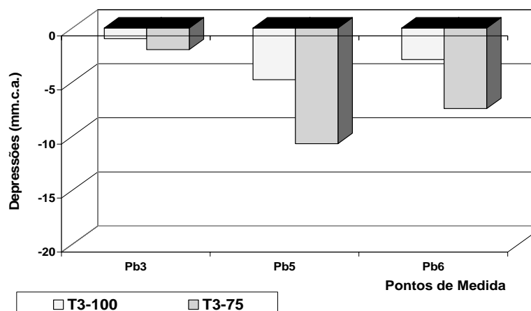
Figura 11 - Depressões máximas no ramo de esgoto da caixa sifonada com arranjo de descarga Da e diâmetros de 100 mm e 75 mm para bacia sanitária com volume de 6,0 litros
