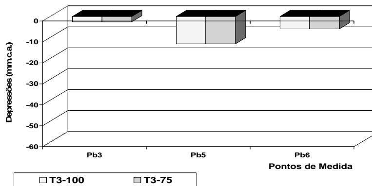
Figura 10 - Depressões máximas no ramo de esgoto da caixa sifonada com arranjo de descarga Da e diâmetros de 100 mm e 75 mm para bacia sanitária com volume de 11,5 litros
