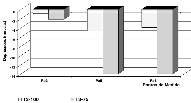
Figura 9 - Depressões máximas no ramo de descarga da bacia sanitária com arranjo de descarga Da e diâmetros de 100 mm e 75 mm para bacia sanitária com volume de 6,0 litros
