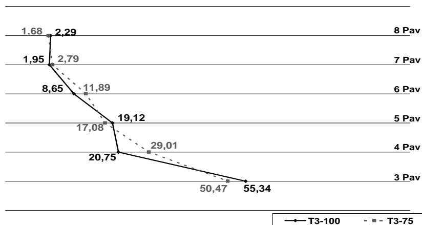
Figura 13 - Pressões positivas máximas, em mm.c.a., no tubo de queda para o arranjo de descarga Da e diâmetros de 100 mm e 75 mm para bacia sanitária com volume de 6,0 litros
