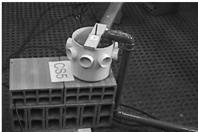
Figura 2 - Alimentação da caixa sifonada nos protótipos
