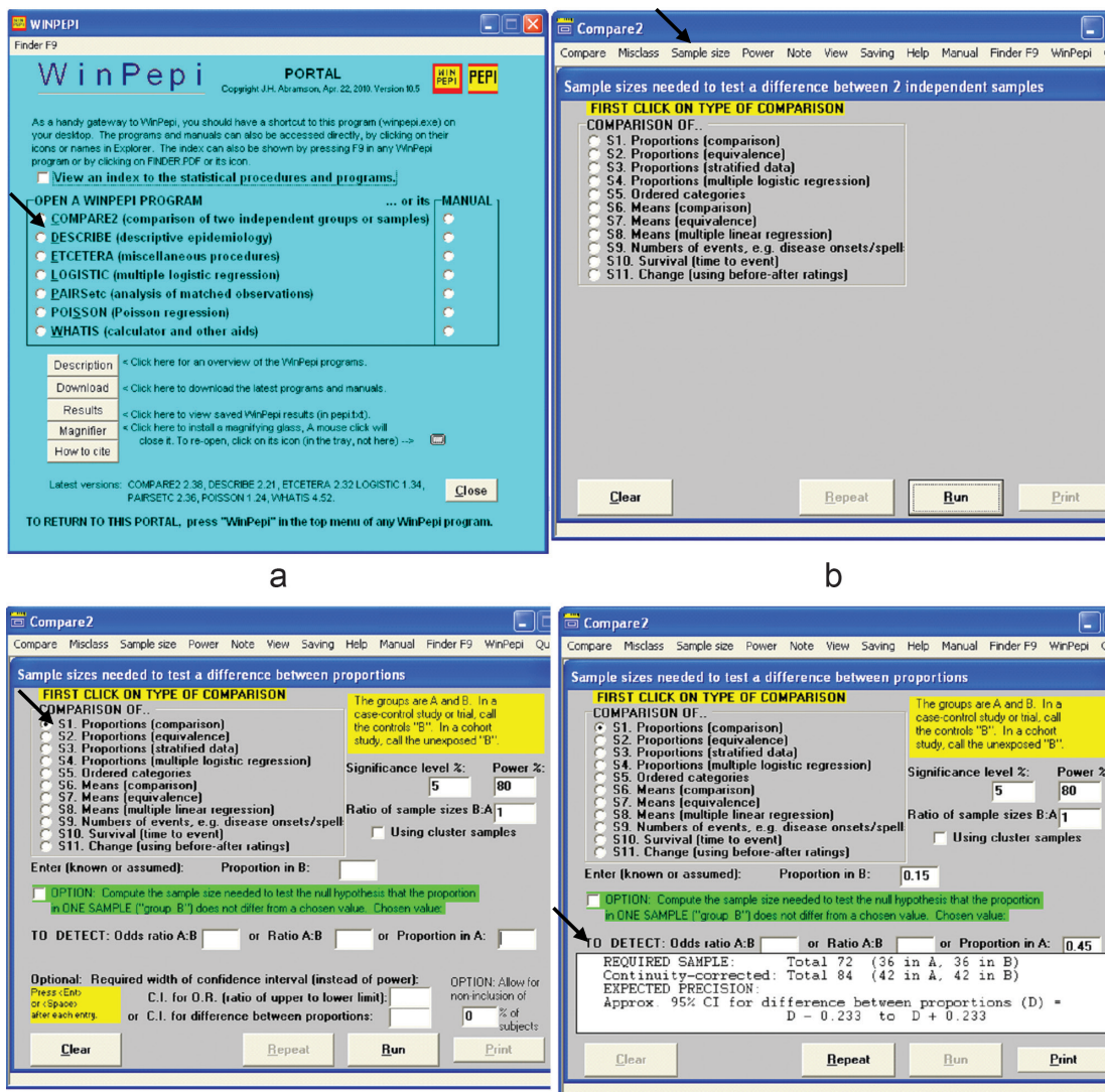
Figura 3: Cálculo do tamanho de amostra para comparação de 2 proporções no programa WINPEPI (versão 10.5).
