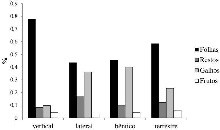
Figura 2. Percentual de folhas, galhos, frutos e restos vegetais na formação dos diferentes compartimentos de aporte de detritos para o riacho Cachoeira Grande medidos entre ago/2010 a ago/2011.
