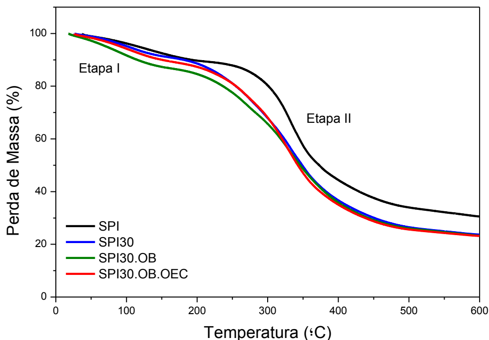
Figura 10. Curva termogravimétrica para os diferentes filmes na taxa de aquecimento de 10\text{ }^{\circ}\text{C min}^{-1} e fluxo de nitrogênio constante ( 50\text{ mL min}^{-1} )
