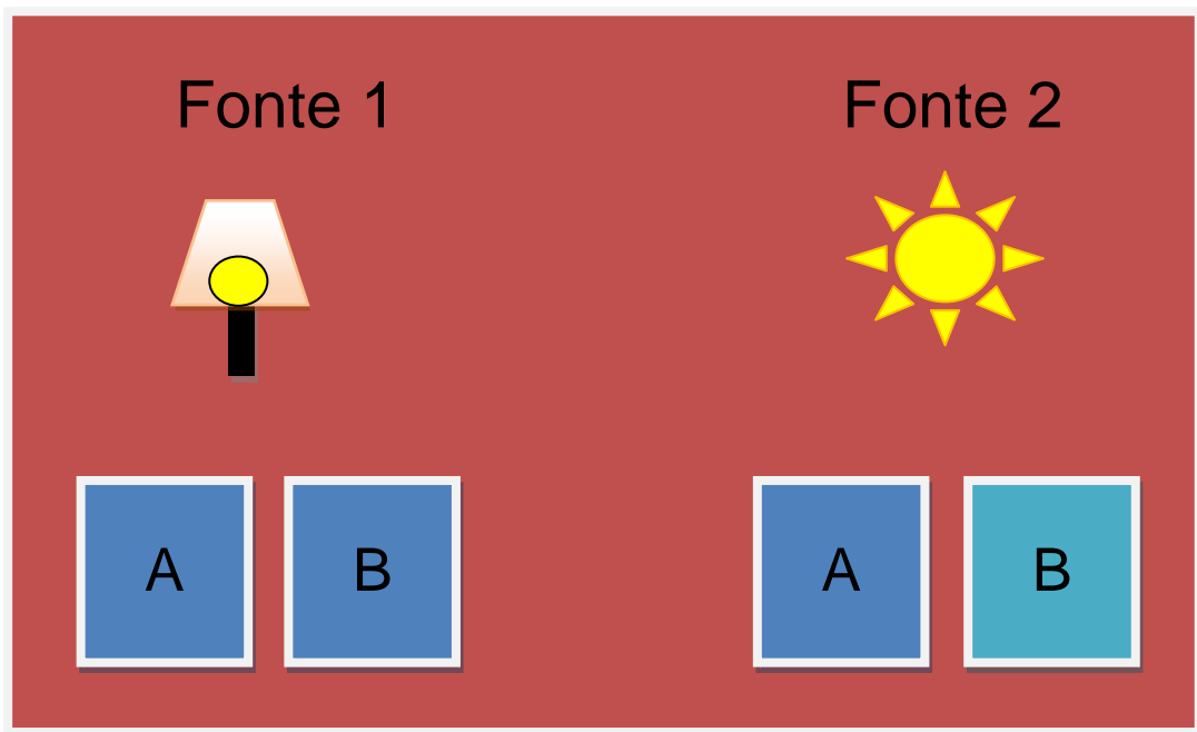
FIG. 2: Metamerismo
