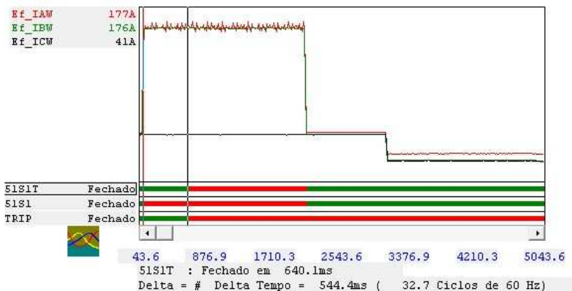
Figura 5.35: Registro oscilográfico da atuação da função 51 para uma falta bifásica (barra 816) no alimentador com GD e grupo de ajuste 2 ativado.
