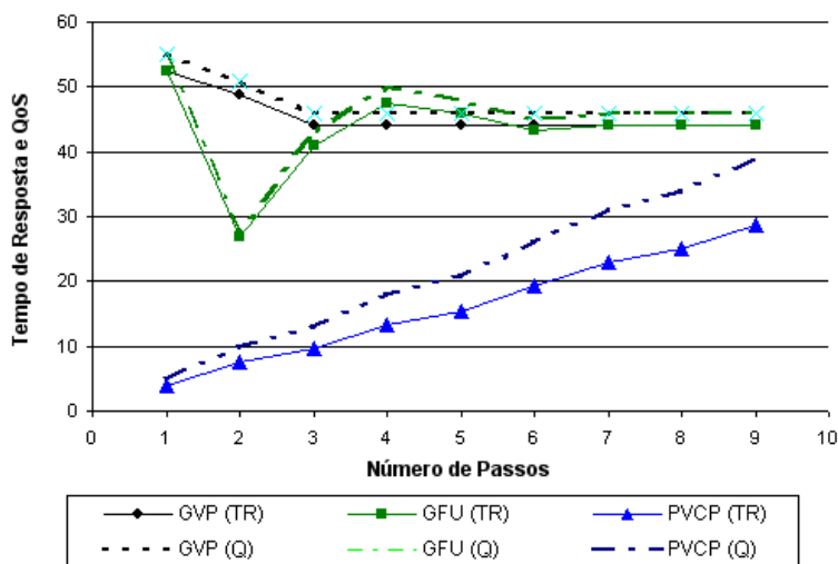
Figura 6.13. Desempenho das heurísticas considerando o Deadline Folgado 45
