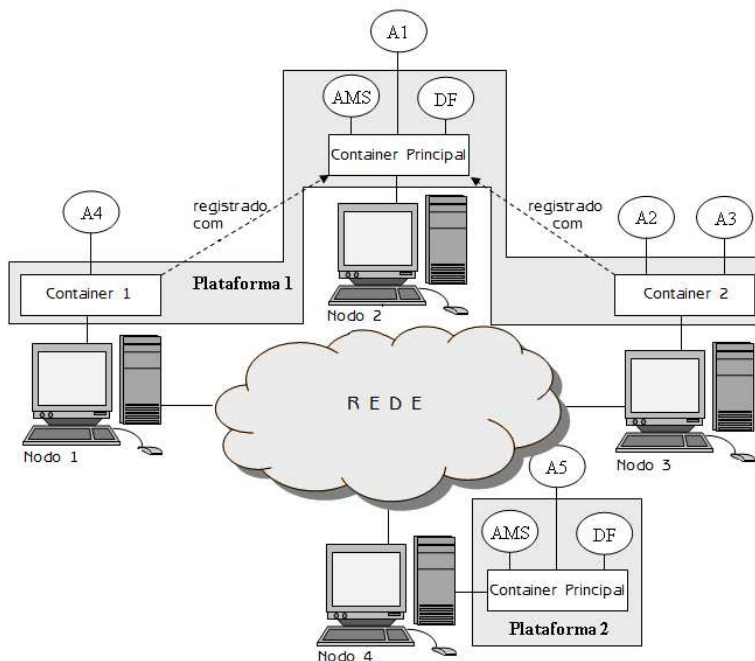
Figura 2.2. A Arquitetura JADE [Bellifemine 2001]
