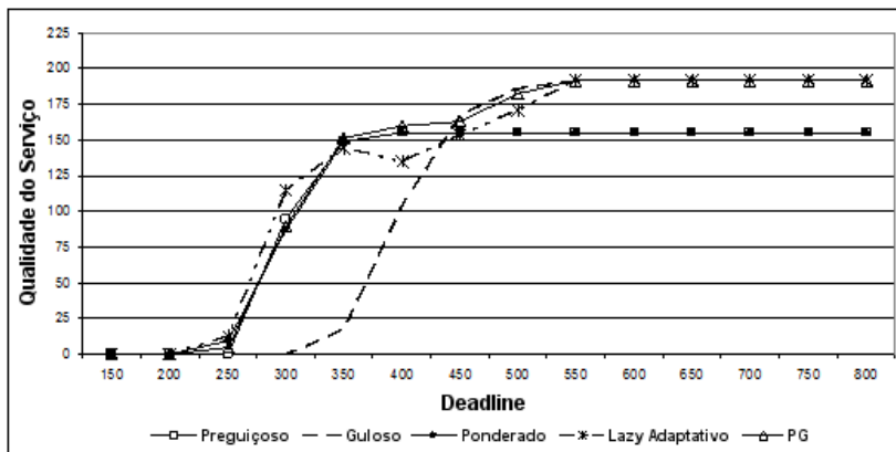
Figura 5.5. Qualidade Global das Heurísticas.
