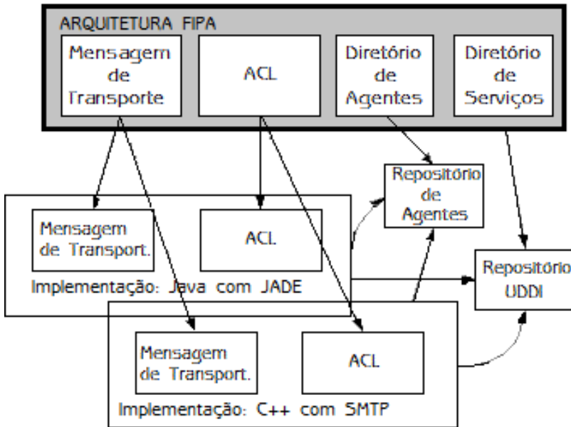
Figura 2.1. Abstração de Arquitetura FIPA [FIPA 2002]
