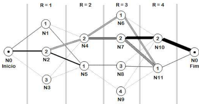
Figura 5.4. Viagens consecutivas com a heurística Lazy-Adaptativo.
