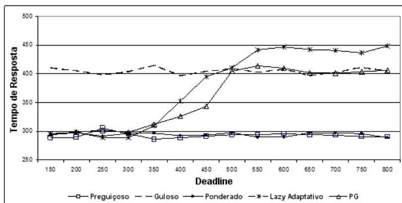
Figura 5.6. Tempo Médio de Resposta das Heurísticas.
