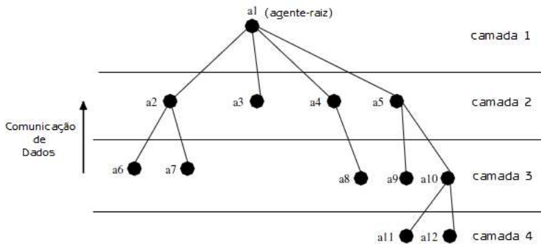
Figura 2.3. Arquitetura em Níveis [Ilarri 2008]
