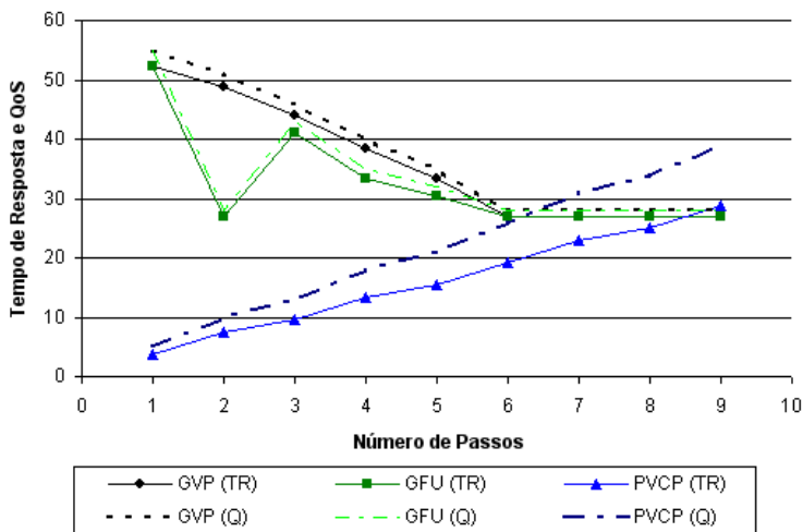
Figura 6.12. Desempenho das heurísticas considerando o Deadline Justo 30
