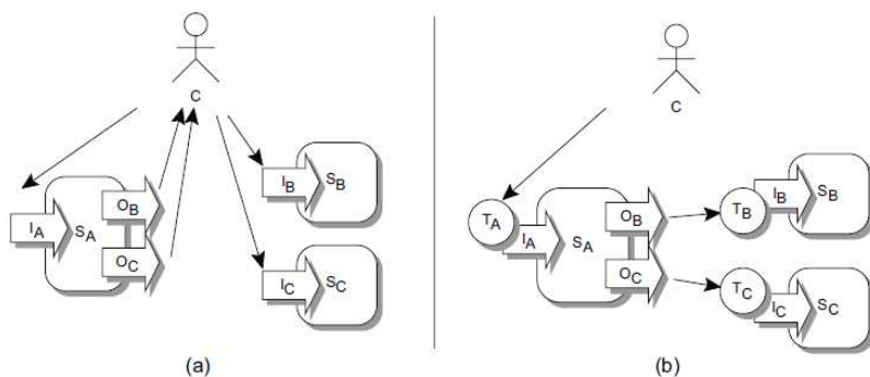
Figura 4.1. Arquitetura baseada em Triggers [Binder 2006]
