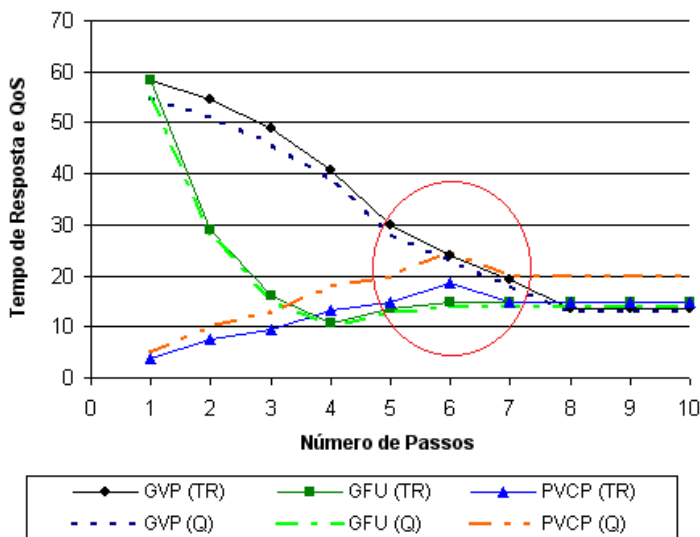
Figura 6.10. Desempenho das heurísticas considerando o Deadline 15 para a missão M1
