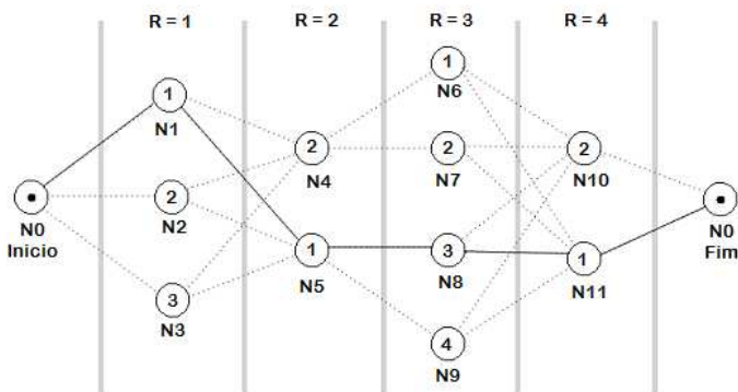
Figura 5.3. Primeira viagem com Lazy-Adaptativo.
