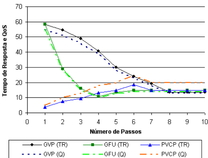
Figura 6.11. Desempenho das heurísticas considerando o Deadline 15 para a missão M2
