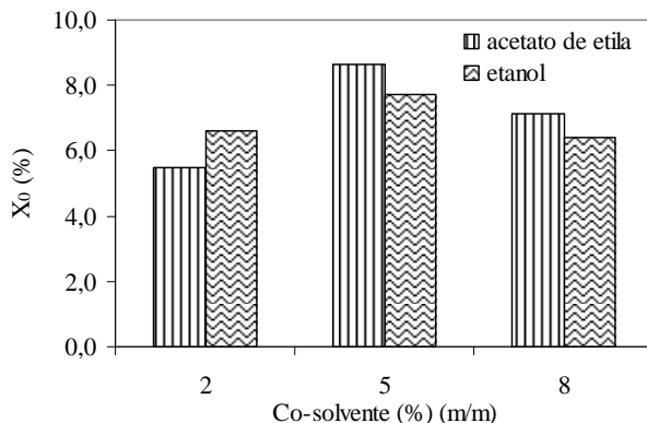
Figura 8: Efeito da concentração e do tipo de co-solvente no rendimento da ESC de erva baleeira.
