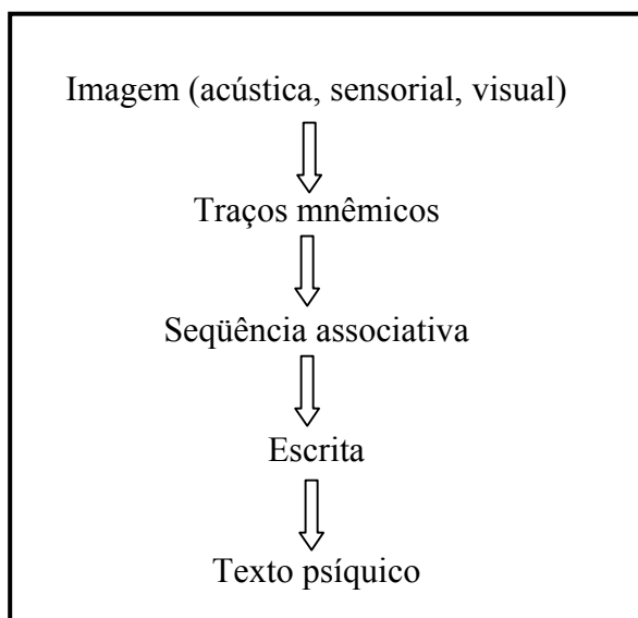
Figura 02 – Aparelho psíquico
