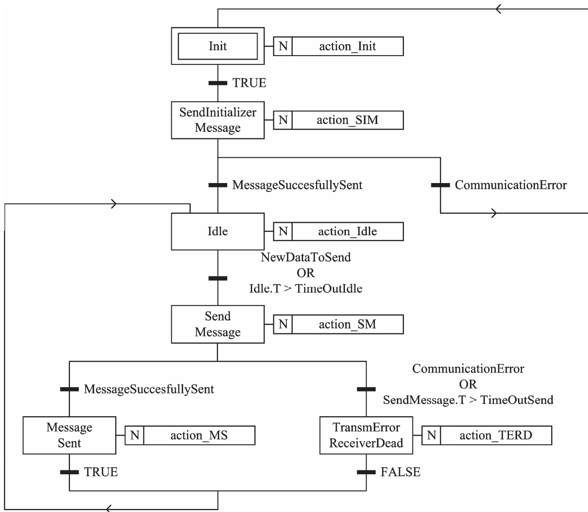
Figura 6.3 – SFC Sender
