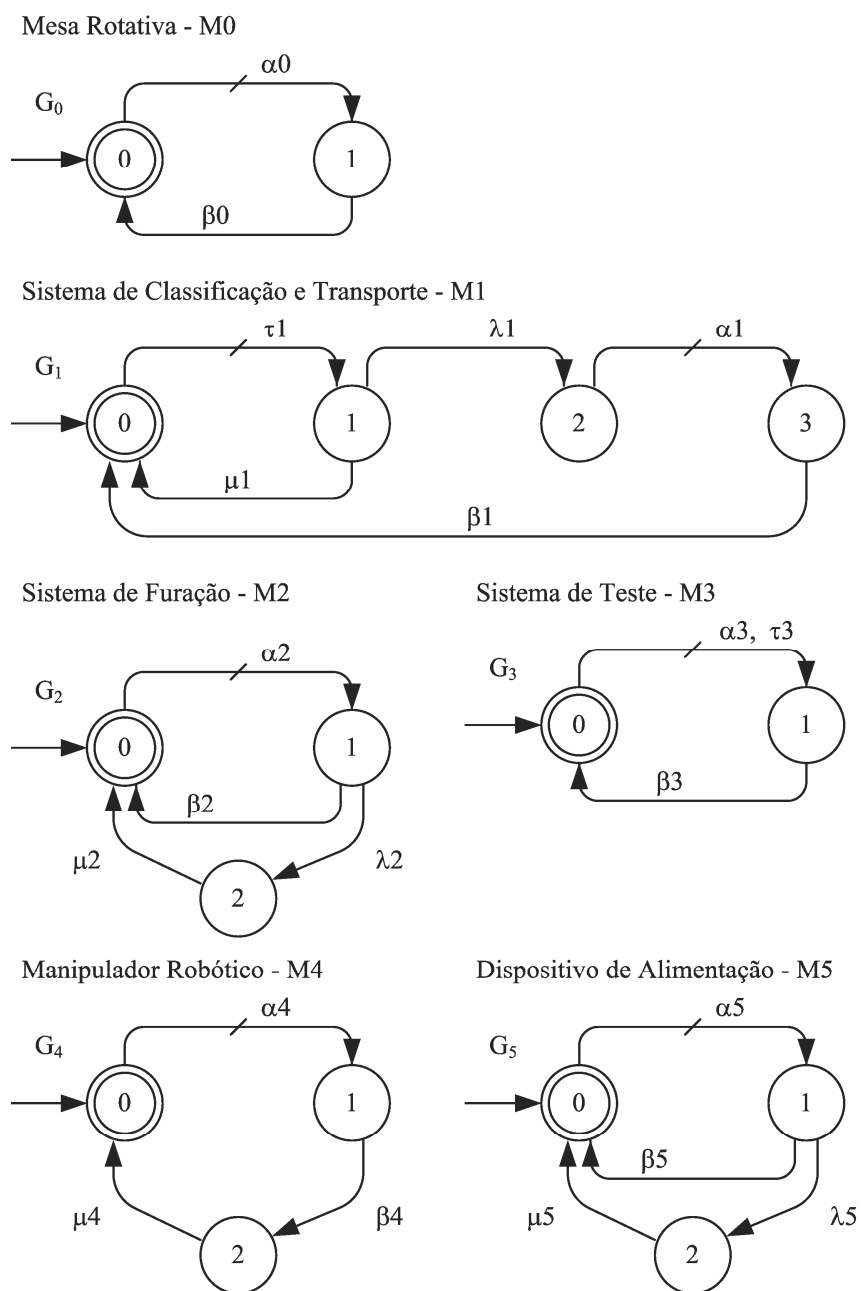
Figura 3.4 – Conjunto de autômatos representando o comportamento independente dos subsistemas que constituem a célula de manufatura
