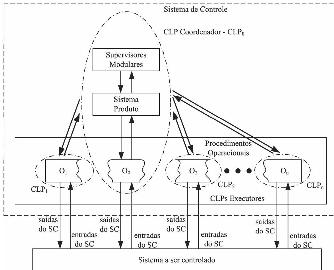
Figura 7.1 – Arquitetura de controle distribuída em múltiplos CLPs
