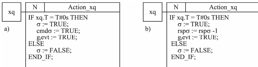
Figura 5.3 – Ações associadas ao passo xq do SFC g_i , i \in I
