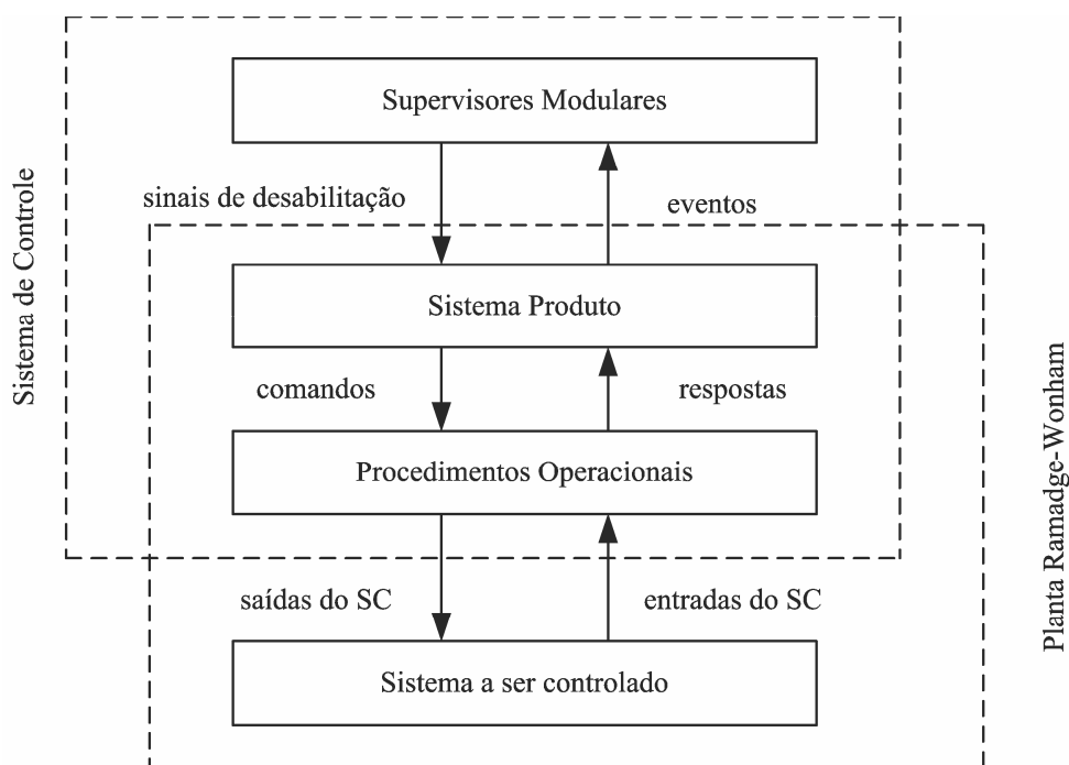
Figura 4.13 – Arquitetura de controle supervísório segundo QUEIROZ e CURY
