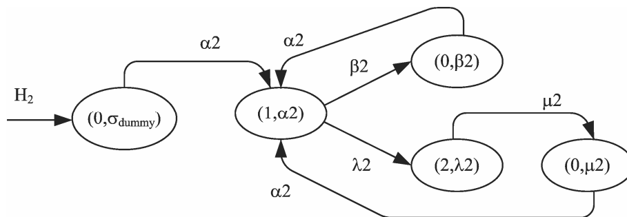
Figura 5.4 – Autômato \mathbf{H}_2 correspondente ao autômato \mathbf{G}_2
