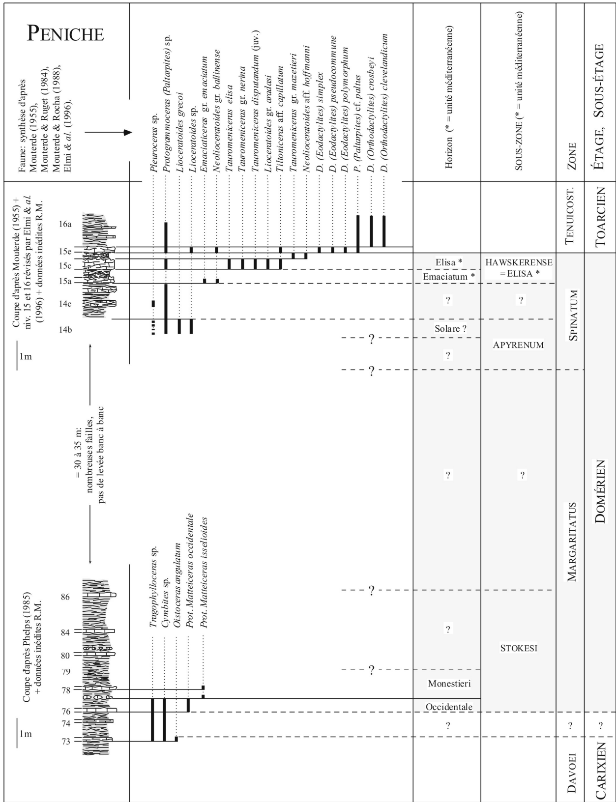
Fig. 5 – Coupe de Peniche avec indication des distributions des ammonites et du cadre biostratigraphique.
