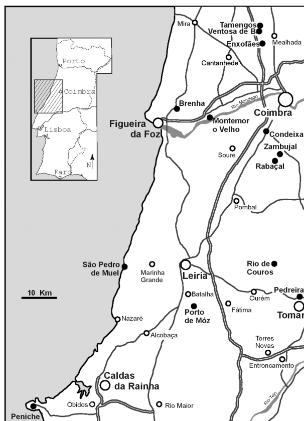
Fig. 2 – Localisation des principaux gisements (caractères gras et points noirs) du Bassin Lusitanien qui ont livré les faunes domériennes étudiées dans le présent travail.
