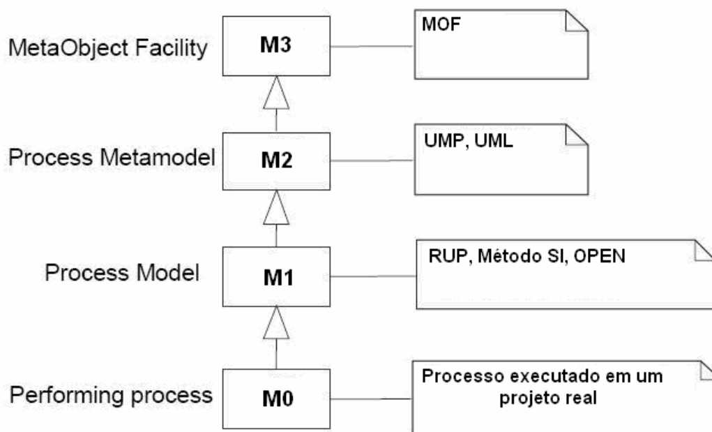
Figura 3: Níveis de Modelagem na arquitetura de quatro camadas da UML (OMG, 2005a).
