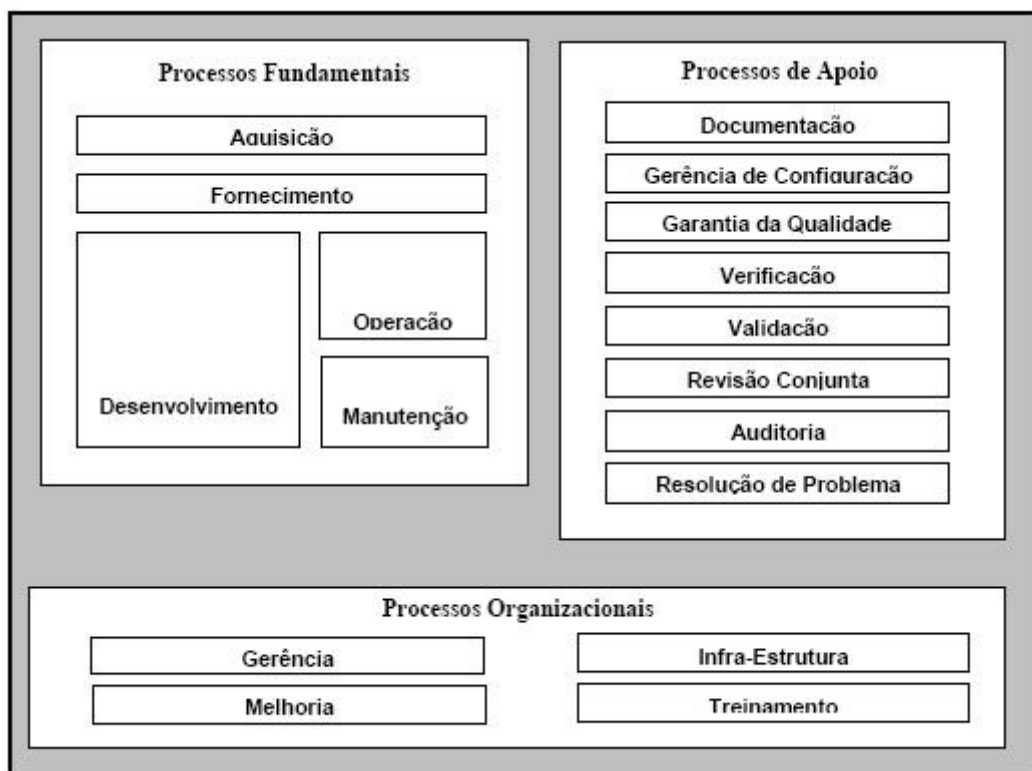
Figura 1: Processos de Software segundo a norma NBR ISO/IEC 12207 (ABNT, 1998).
