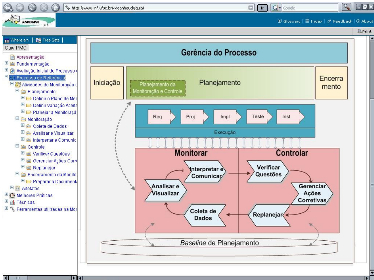
Figura 42: Processo de Referência para Monitoramento e Controle em alto nível.
