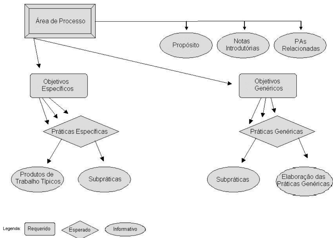
Figura 14: Estrutura básica do CMMI-DEV V 1.2 (SEI, 2006)
