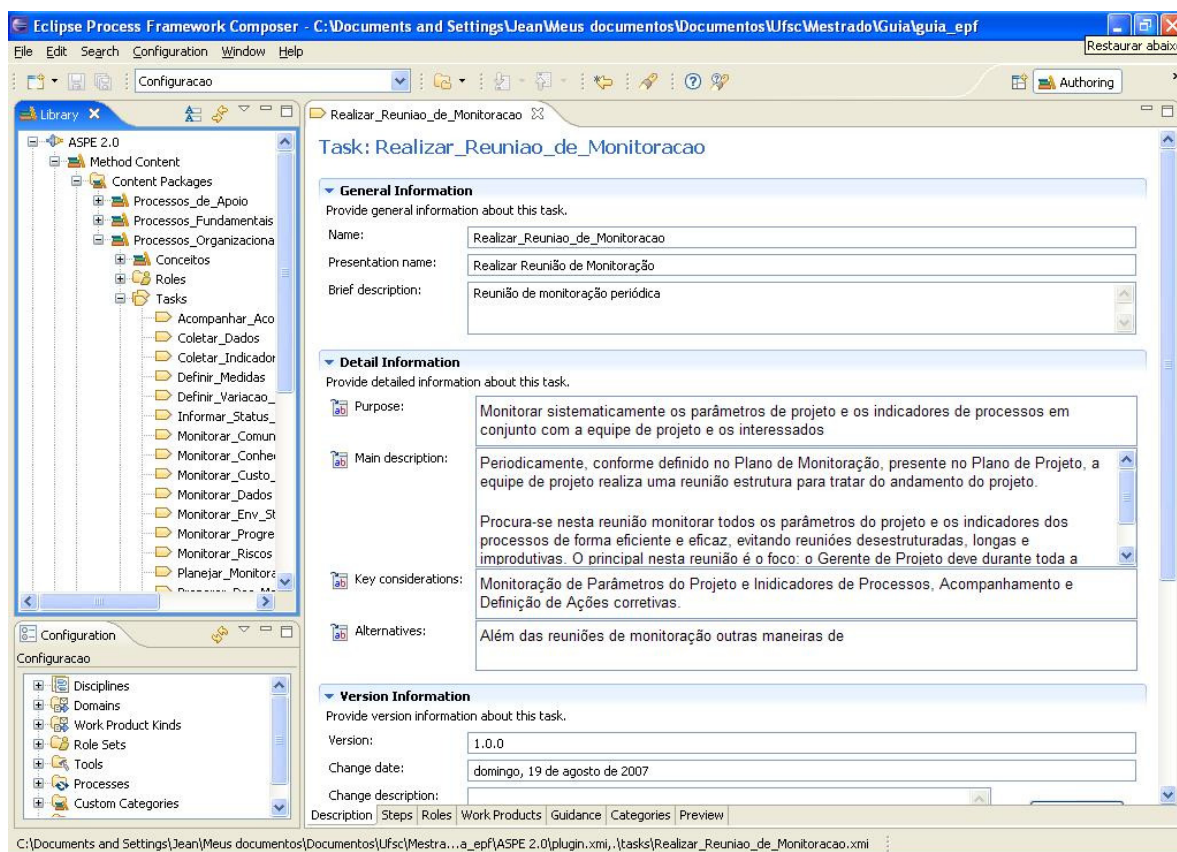
Figura 37: Registro do Guia de Referência no Eclipse Process Framework .
