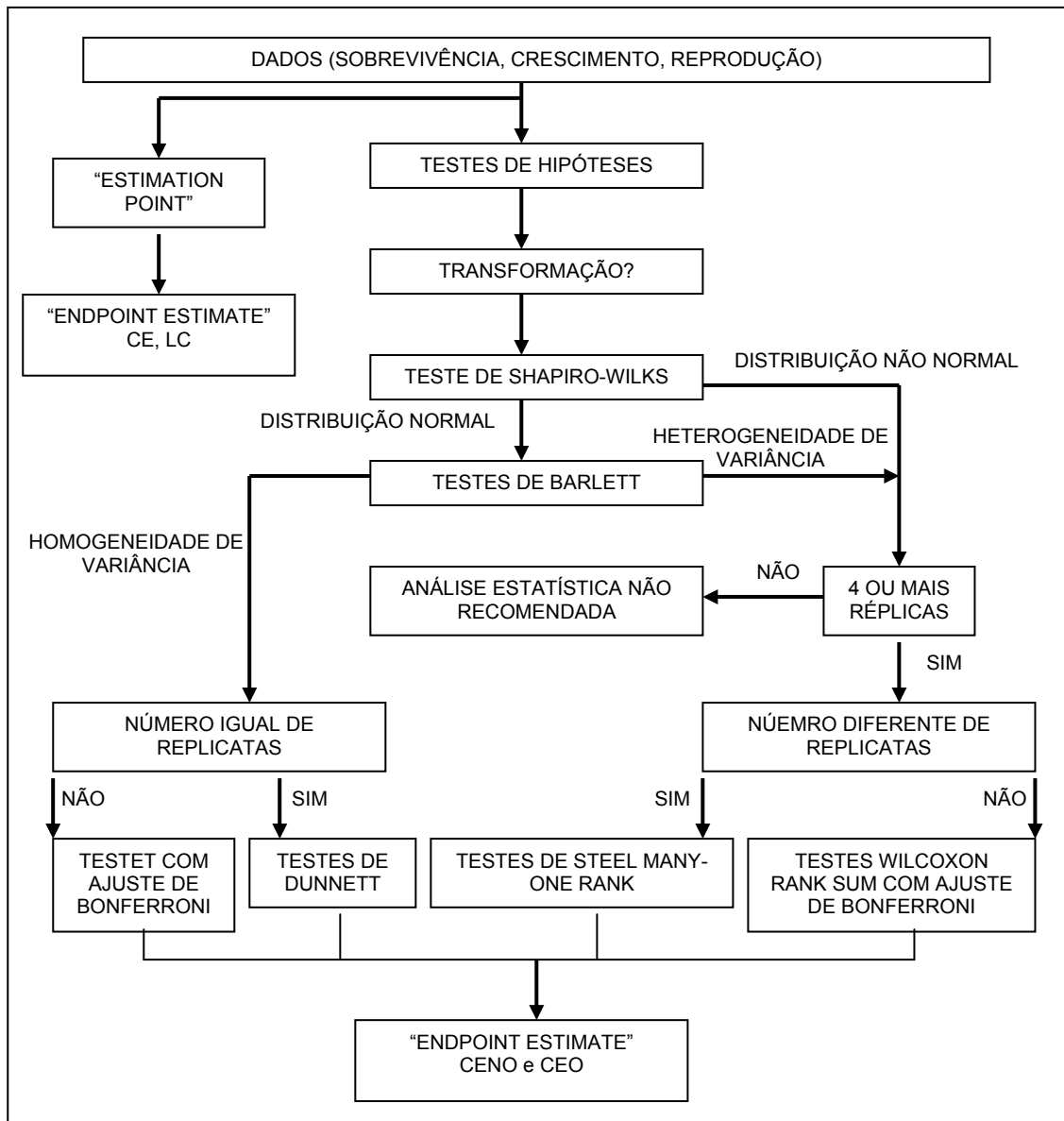
FIGURA 13: Fluxograma para análise estatística de dados.
