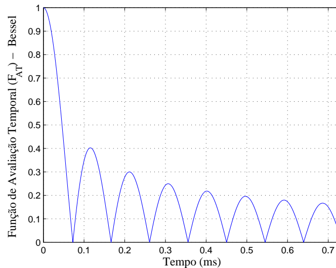
Figura 4.3: Função de avaliação temporal quando o transmissor possui o conhecimento da velocidade do usuário no esquema TC-OBF. Para esta figura consideramos v = 3 km/h, f_c = 1,9 GHz e time slot com 1,67 ms de duração.
