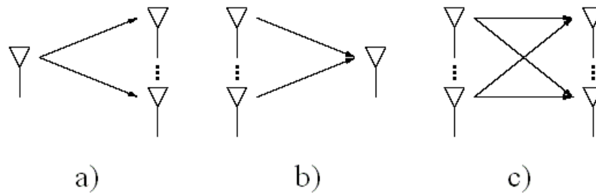
Figura 2.5: Configuração de antenas para diversidade espacial. a) Diversidade de recepção (SIMO); b) Diversidade de transmissão (MISO); c) Diversidade de transmissão e recepção (MIMO).
