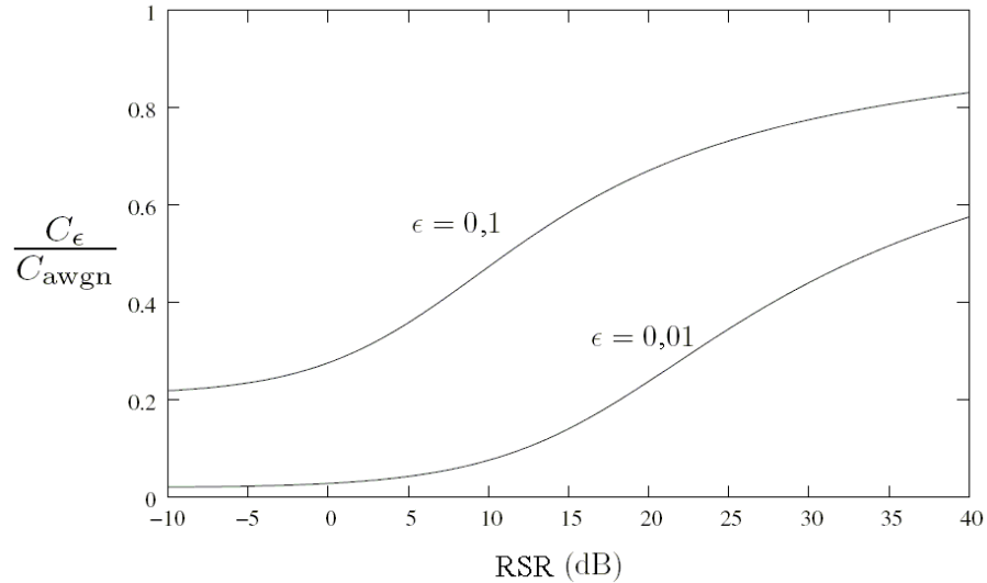
Figura 2.8: Comparação entre a capacidade dos canais AWGN e a capacidade de interrupção para canais com desvanecimento lento para \epsilon = 0,1 e \epsilon = 0,01 . Modificada de (TSE; VISWANATH, 2005).
