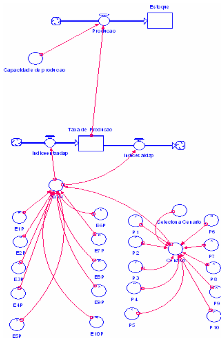
Figura 7.2: Modelo de simulação para Cenários Prospectivos através da modelagem hard da Dinâmica de Sistemas
