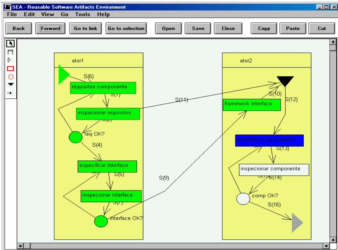
Figura 20– Atividade especificar componente, em andamento
