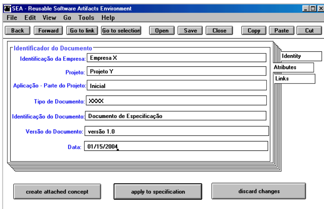
Figura 7.9 - Janela de edição do conceito identificador do documento
