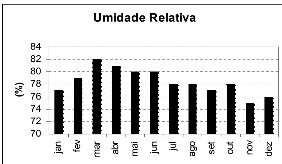
Figura 4 – Umidade Relativa mensais para Caxias do Sul de 1961 a 1990 Fonte: Normas climatológicas – INMET.
