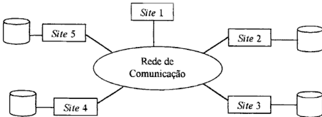
Figura 1 - Banco de dados distribuído
