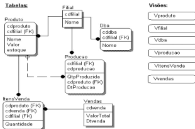
Figura 10 - Modelo de dados dos sítios (antes da distribuição dos dados)
