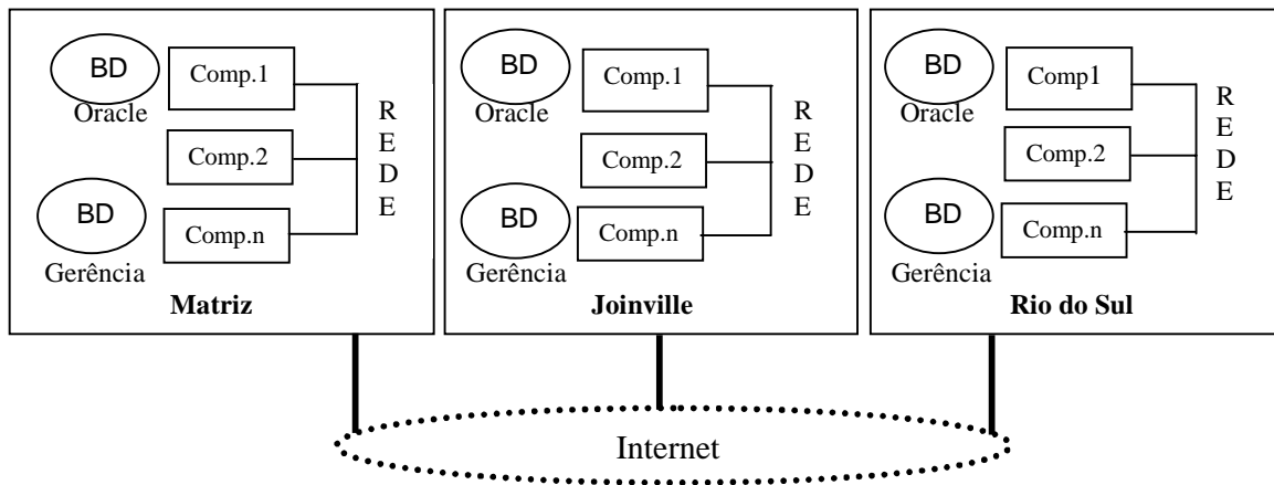
Figura 9 - Ambiente de implementação
