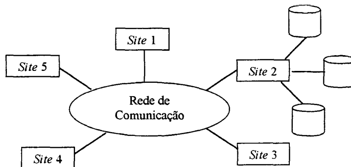
Figura 2 - Banco de dados centralizado em uma rede de computadores
