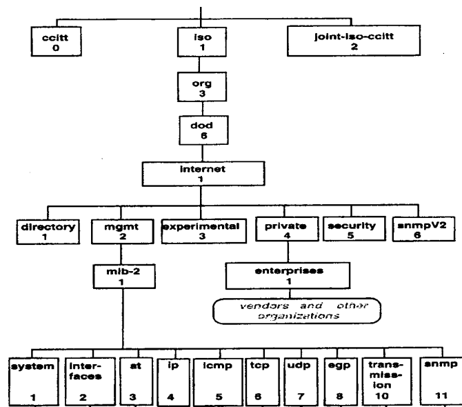
Figura 6 - Árvore de identificadores de objetos
