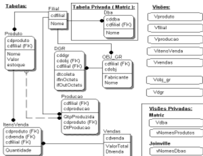
Figura 11 - Modelo de dados dos sítios (depois da distribuição dos dados)
