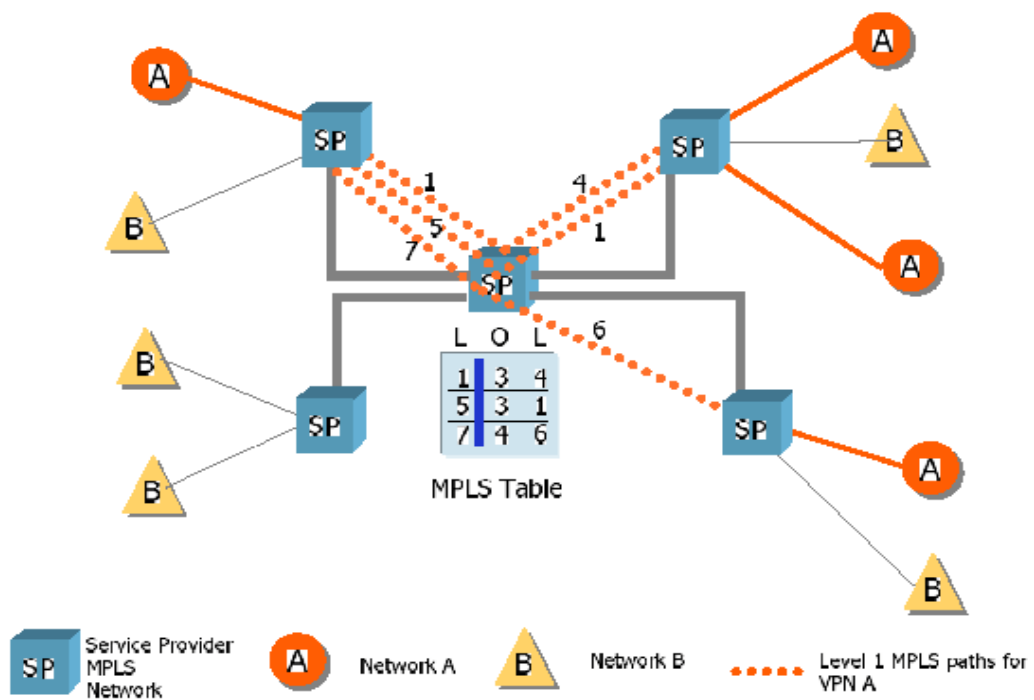
Figura 3 – Estrutura MPLS
