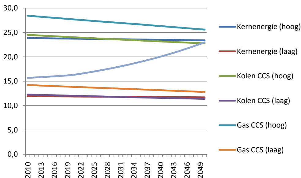
Figuur 4.17 Kostencurven productiekosten fossiel, in € mln per PJ
