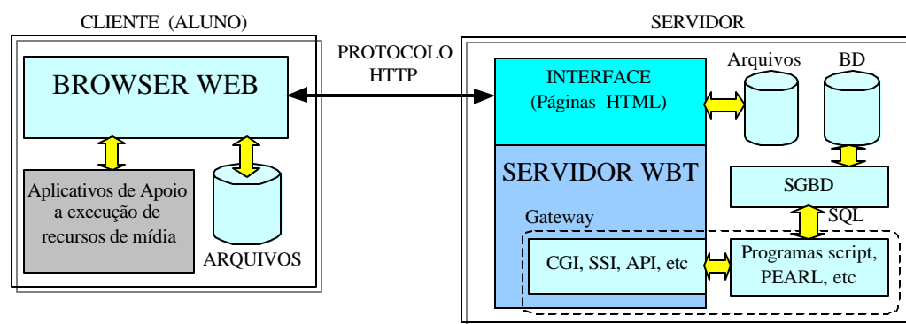
Figura 8 – Arquitetura cliente-servidor que compõe cada interface do modelo
