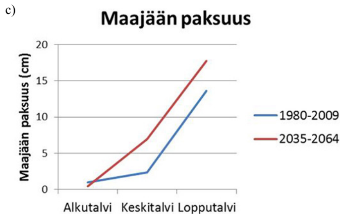
Kuva L-3. Keskimääräinen avoimen ympäristön lumen syvyyden maksimi (a), lumen tiheys (b) ja maajään paksuus (c) kontrollijakson (1980-2009) ja skenaariojakson (2035-2064) aikana Sodankylässä. Sodankylän säähavaintoaseman havaintoja käytettiin kuvaamaan keskimääräisiä Metsä-Lapin oloja. Alkutilvella tarkoitetaan ajanjaksoon 1.10-15.12, keskitalvella 16.12-28.2 ja lopputilvella 1.3-15.5 (Turunen et al. 2015a,b).
