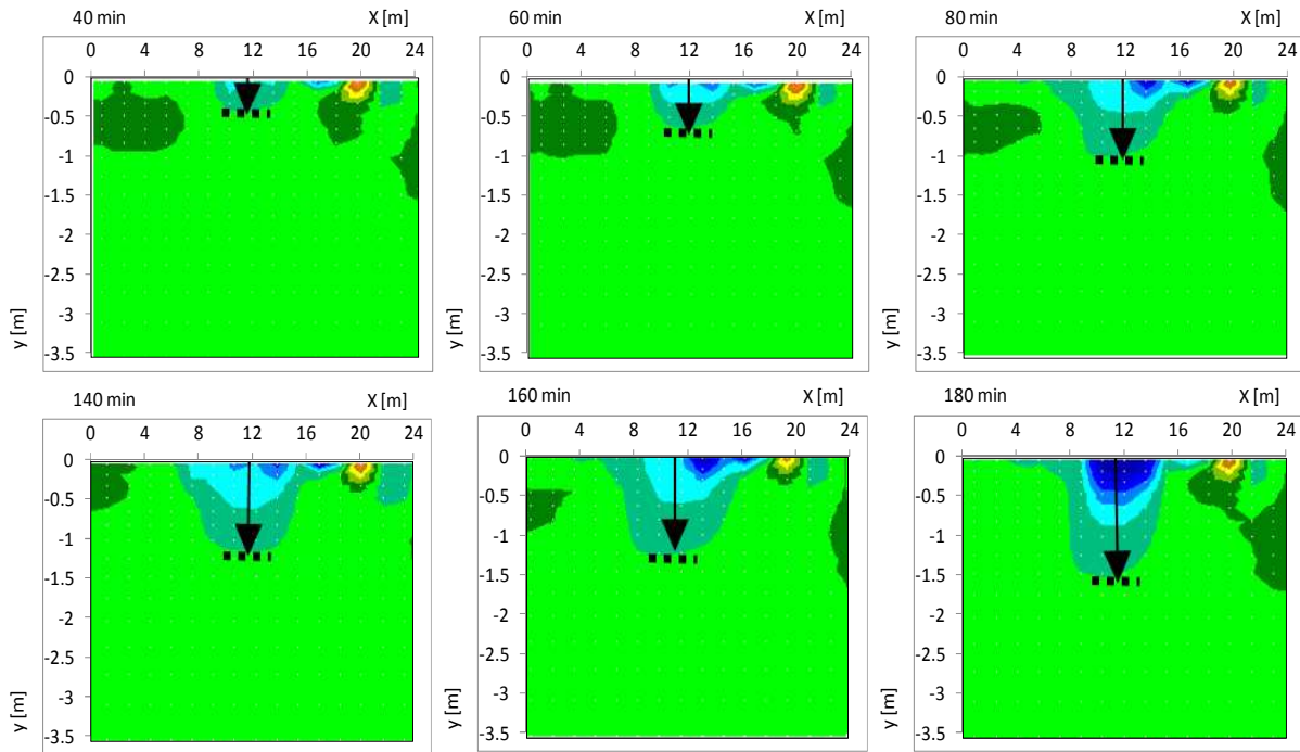
Figure 6. Tomographie électrique time lapse : différences de résistivité dans les différents instants de temps par rapport à la valeur du terrain non perturbé. La ligne pointillée indique le front d'infiltration.
