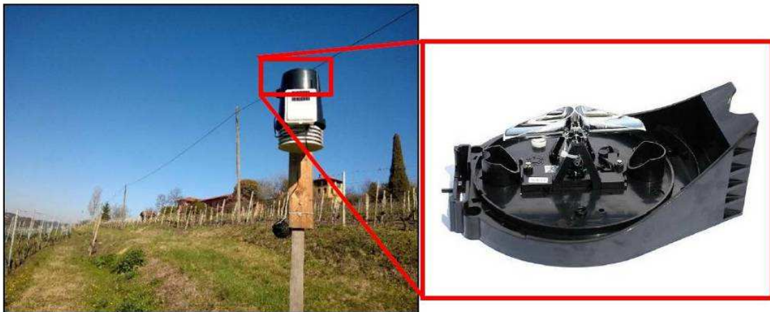
Figure 2. Pluviomètre à bascule installé sur le côté d'étude. Encadré en rouge le détail de l'instrument.
