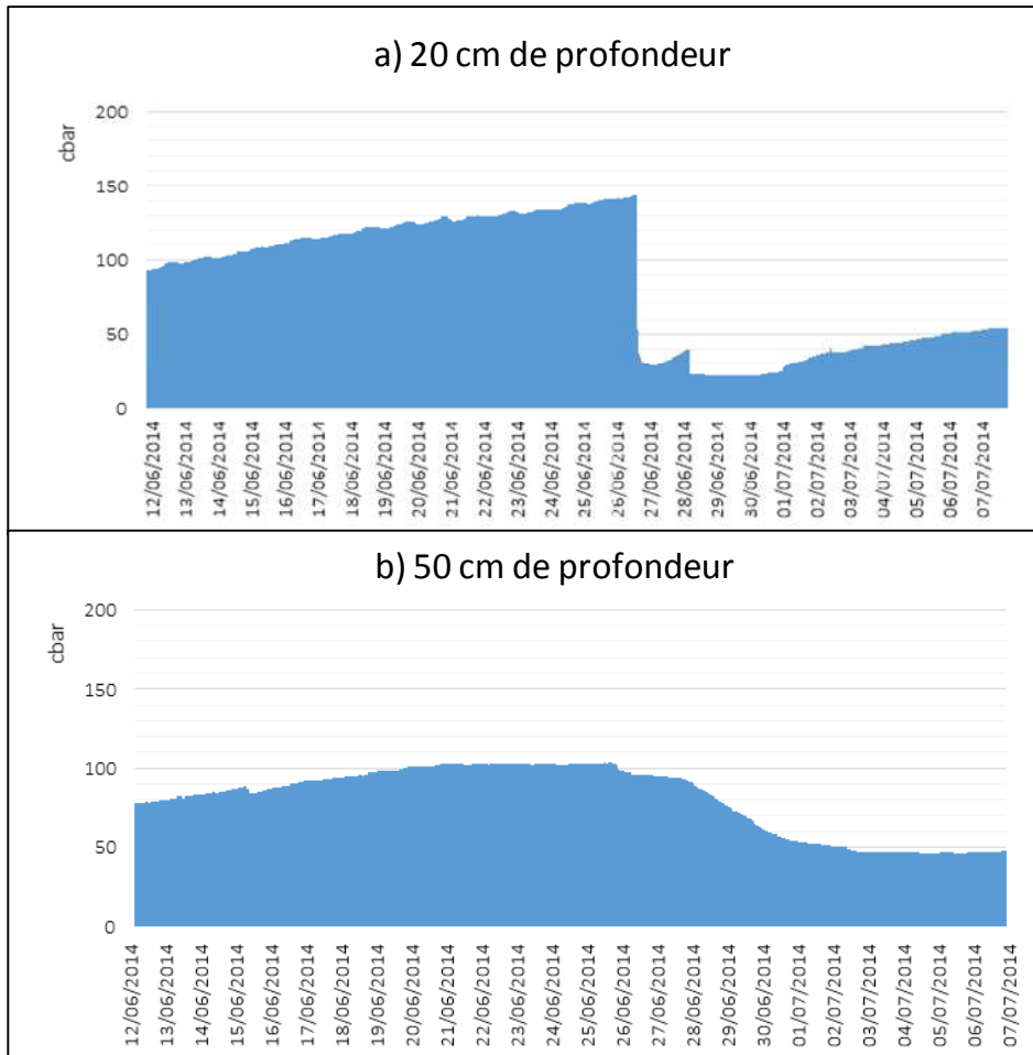
Figure 5. Mesures des tensiomètres du 12/06/2014 au 07/07/2014: a) à 20 cm de profondeur, b) à 50 cm de profondeur.
