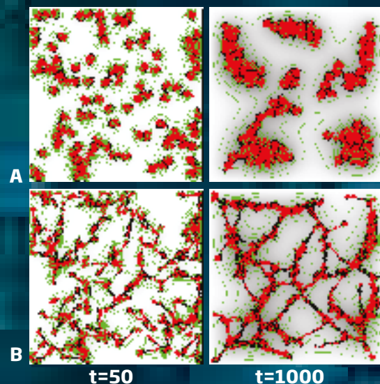
Figuur 1: Simulatie van cellen die elkaar aantrekken met een groeifactor. A. Cirkelvormige cellen; B. Langgerekte cellen. Cellen weergegeven in rood, celgrenzen zwart; grijstinten: concentratie groeifactor; groene curves: contourlijnen van concentratie groeifactor. Tijd in Monte Carlo steps, de gebruikelijke tijdstap in Cellular-Potts-simulaties. Voor details zie Ref. [5].
