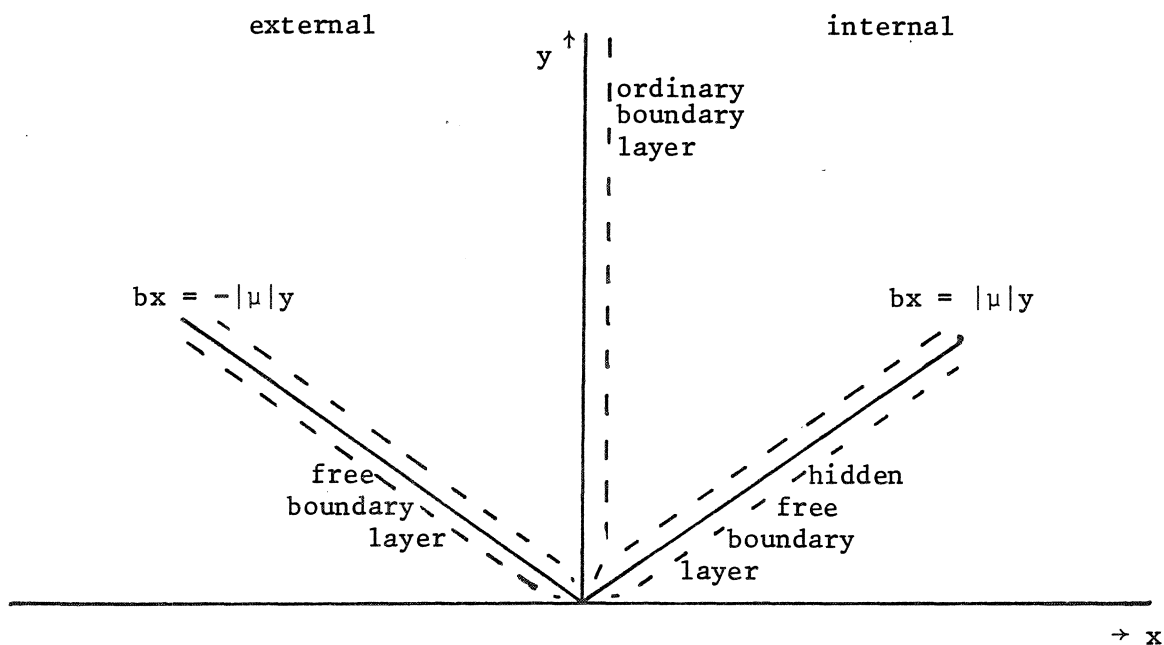
fig. 1 : \mu < 0 .
