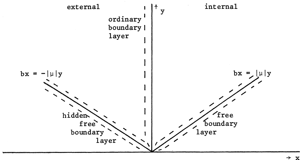
fig. 2 : \mu > 0 .
