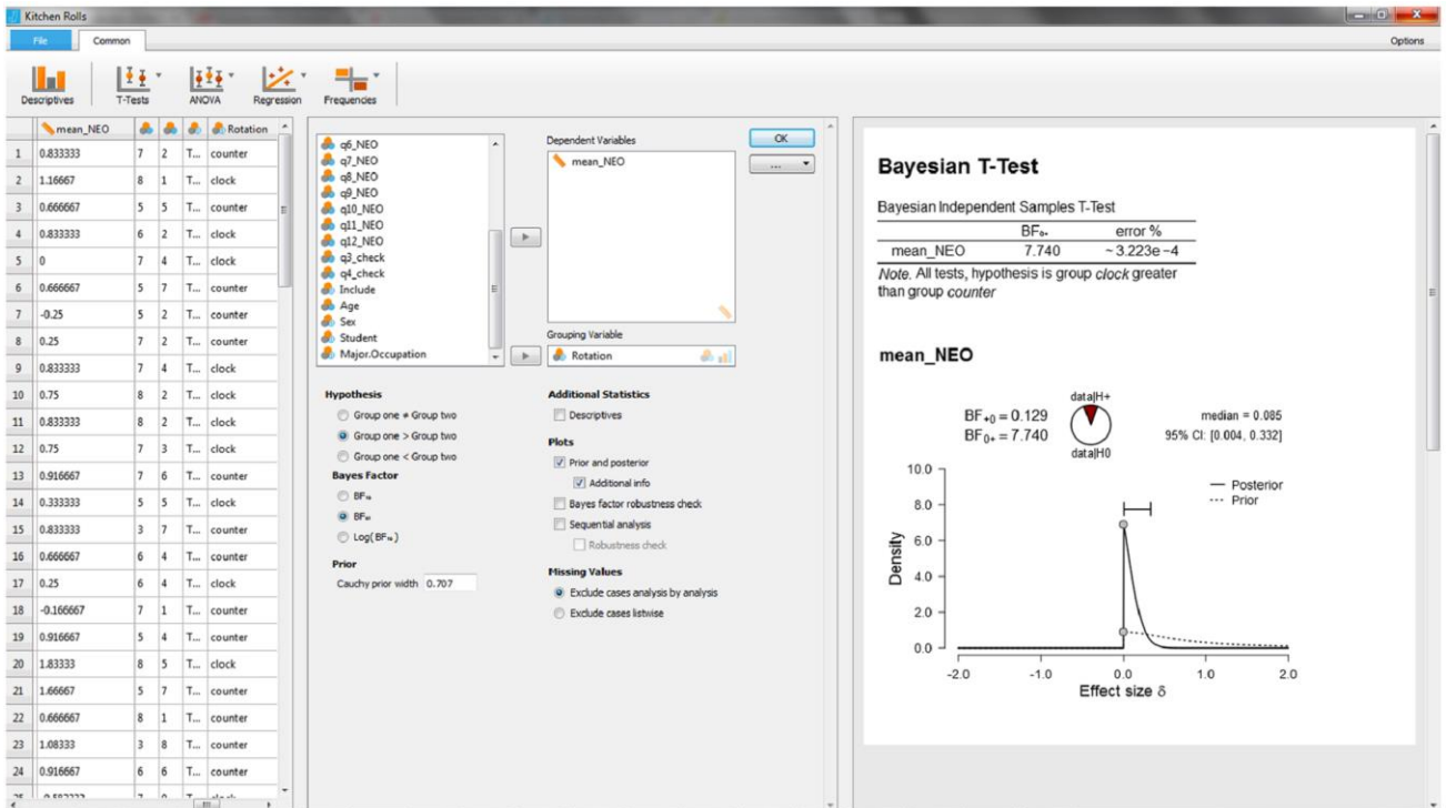
图 3 使用 JASP 对 Wagenmakers 等人(2015) (Wagenmakers, et al., 2015)数据进行贝叶斯单侧独立样本 t 检验的示意图。
