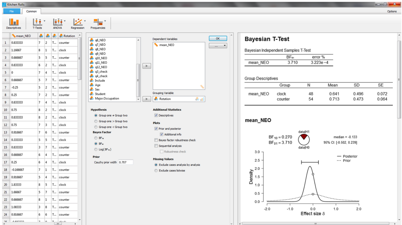
图2 使用 JASP 进行贝叶斯独立样本 t 检验时的操作截屏。软件左侧是数据；中间为数据分析选项；右侧为结果输出。
