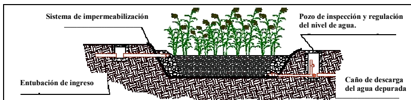
Figura 13: Fitodepuración
