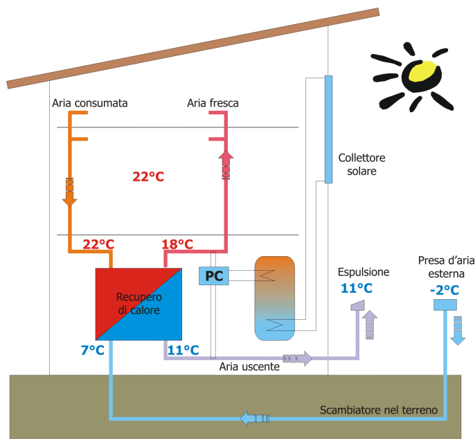
Fig. 5 - Schema di funzionamento di un impianto di ventilazione con recupero calore e scambiatore interrato tipico delle passivhaus italiane (Carletti C. et al, 2004)
