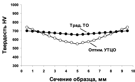
Рис. 2. Распределение твердости HV по сечению образцов из стали Р18 (а) и стали У8 (б), подвергнутых традиционной ТО и оптимальной УТЦО: режим традиционной ТО стали Р18: закалка от 1270 °С + отпуск 560 °С, 1 ч, 3 раза; режим УТЦО стали Р18: ТЦО 1270 °С \leftrightarrow 750 °С, 3 цикла с закалкой + отпуск 560 °С, 1 ч, 3 раза; режим традиционной ТО стали У8: закалка от 790 °С + отпуск 200 °С, 2 ч; режим УТЦО: ТЦО 780 °С \leftrightarrow 230 °С, 4 цикла, с закалкой + отпуск 200 °С, 2 ч. Условия измерения твердости: автоматический прибор «Zwick», нагрузка индентора – 10 Н
