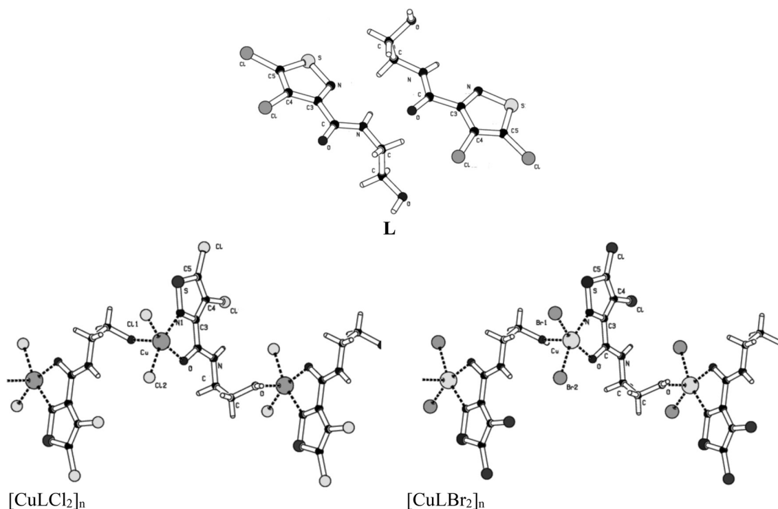
Структуры лиганда L (пара молекул в кристаллической ячейке) и фрагментов полимерных цепочек комплексов [CuLCl 2 ] n и [CuLBr 2 ] n
