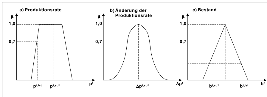
Abbildung 1: Bewertung einer Produktionsrate (a), einer Produktionsänderung (b) und eines Bestandes (c)
