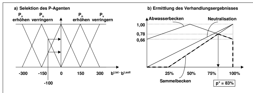
Abbildung 4: Selektion des Verhandlungspartners und Ermittlung des Verhandlungsergebnisses (Schritt 1)
