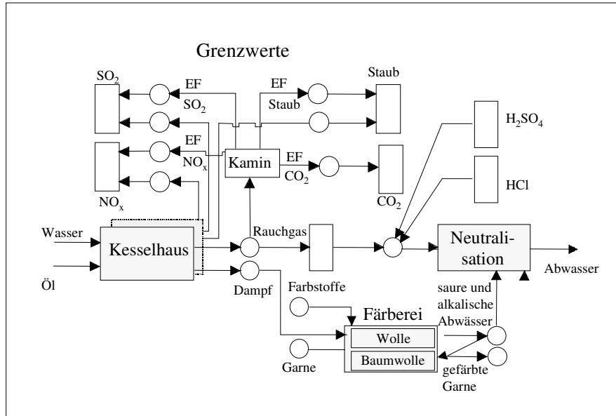
Abbildung 6: Ausschnitt aus dem betrachteten Produktionssystem
