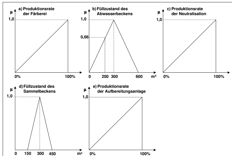
Abbildung 3: Produktionssituation (Ausgangslage)
