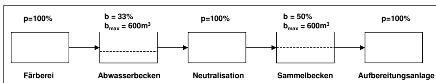
Abbildung 2: Ausschnitt aus dem betrachteten Produktionssystem
