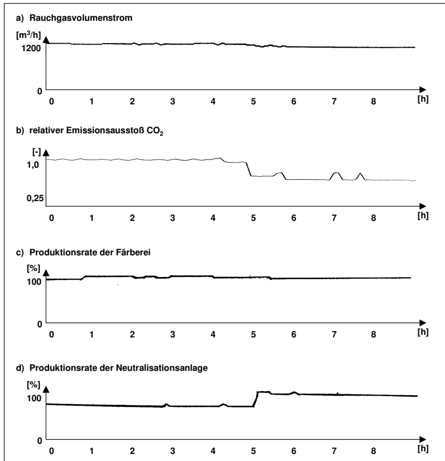
Abbildung 7: Ergebnisse für den betrachteten Systemausschnitt
