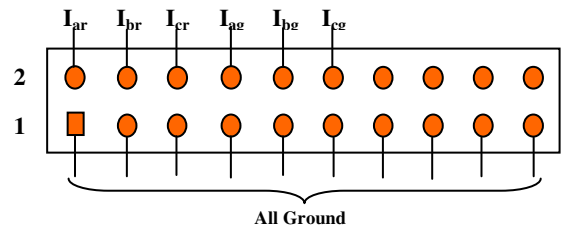
P9 ADC Inputs
