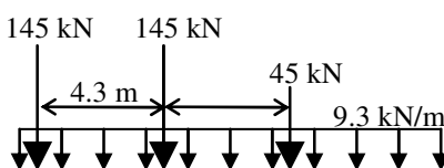
(b) AASHTO live load model (AASHTO-LRFD, 2007);
