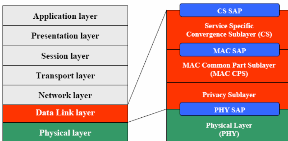
Fig. 2.4. Estructura de protocolos de 802.16.
