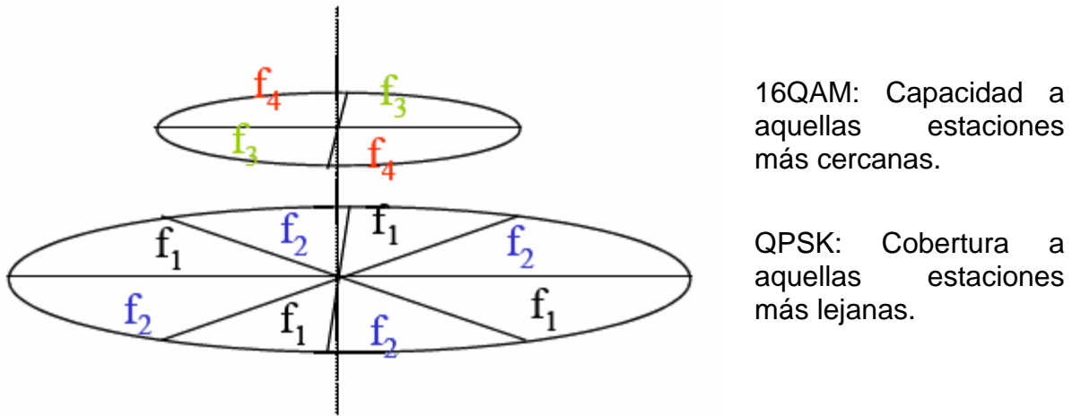
Fig. 1.5. Combinación de las técnicas de modulación adaptativa y sectorización.
