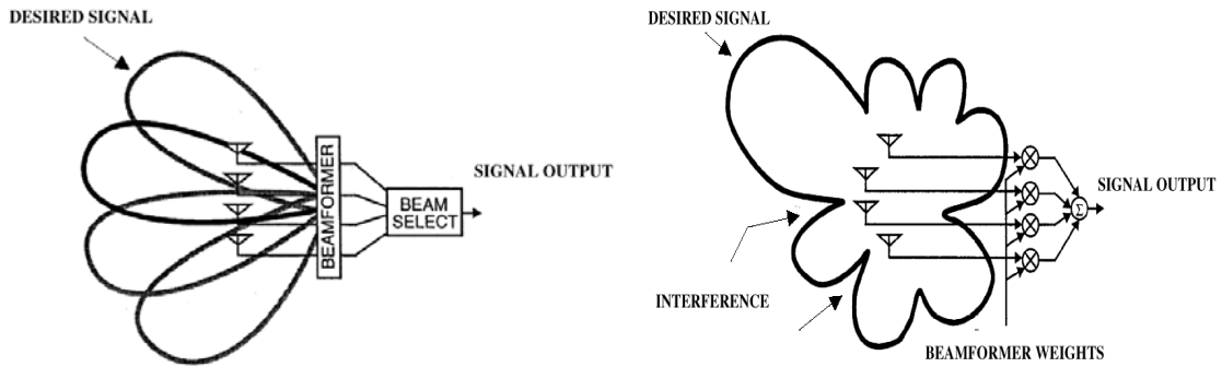
Fig. A2.4. Ejemplo gráfico de antena adaptativa
