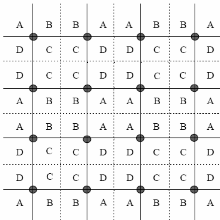
Fig. 1.3. Planificación celular rectangular con sectores de 90^\circ .
