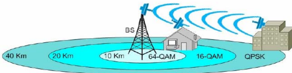
Fig. 2.5. Efectos de la modulación adaptativa.
