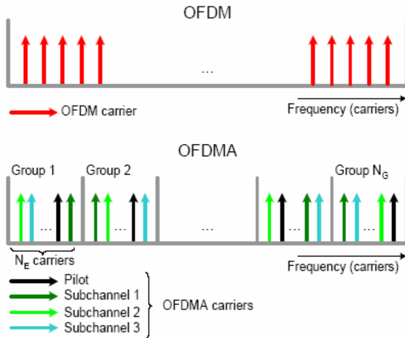
Fig. A2.2. Distribución de las portadoras en modulación OFDM/OFDMA
