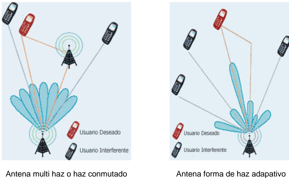
Fig. A2.5. Configuraciones de sistemas AAS
