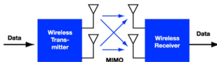
Fig. A2.6. Esquema de un sistema MIMO 2 x 2
