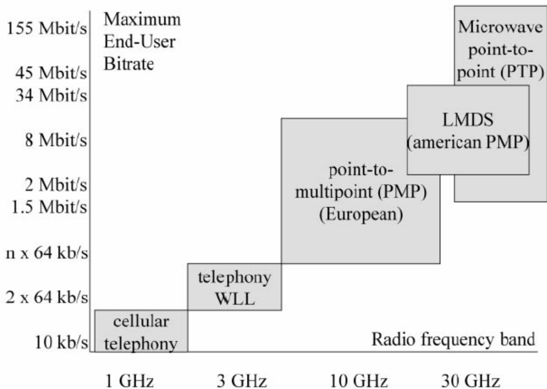
Fig. 1.1. Relación empírica entre la capa radio y el bit rate soportado por el usuario en redes BWA.
