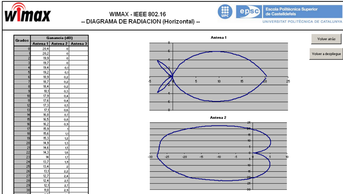
Fig. A1.8. Captura de la pantalla del diagramas de radiación de la herramienta.
