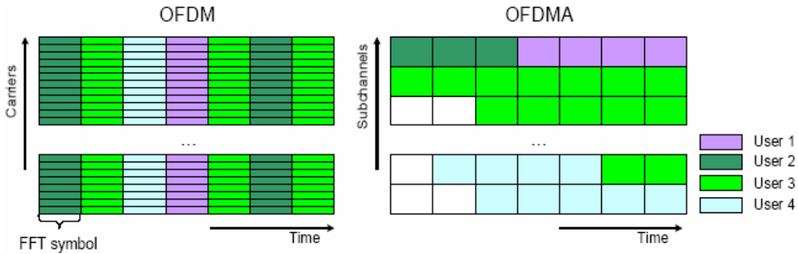
Fig. A2.1. Distribución de los usuarios en modulación OFDM/OFDMA
