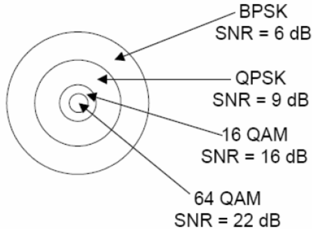
Fig. A2.3. Relación de codificación vs SNR en receptor
