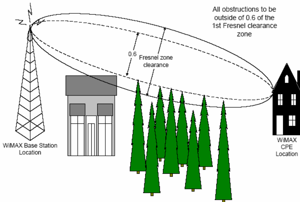
Fig. 2.6. Zona de Fresnel.
