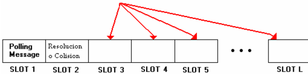
Fig. 2.8 Esquema del CRI
