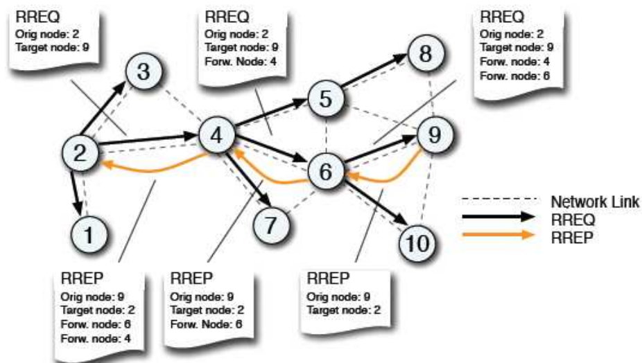
Figura 5.12 Descubrimiento de rutas en el protocolo DYMO
