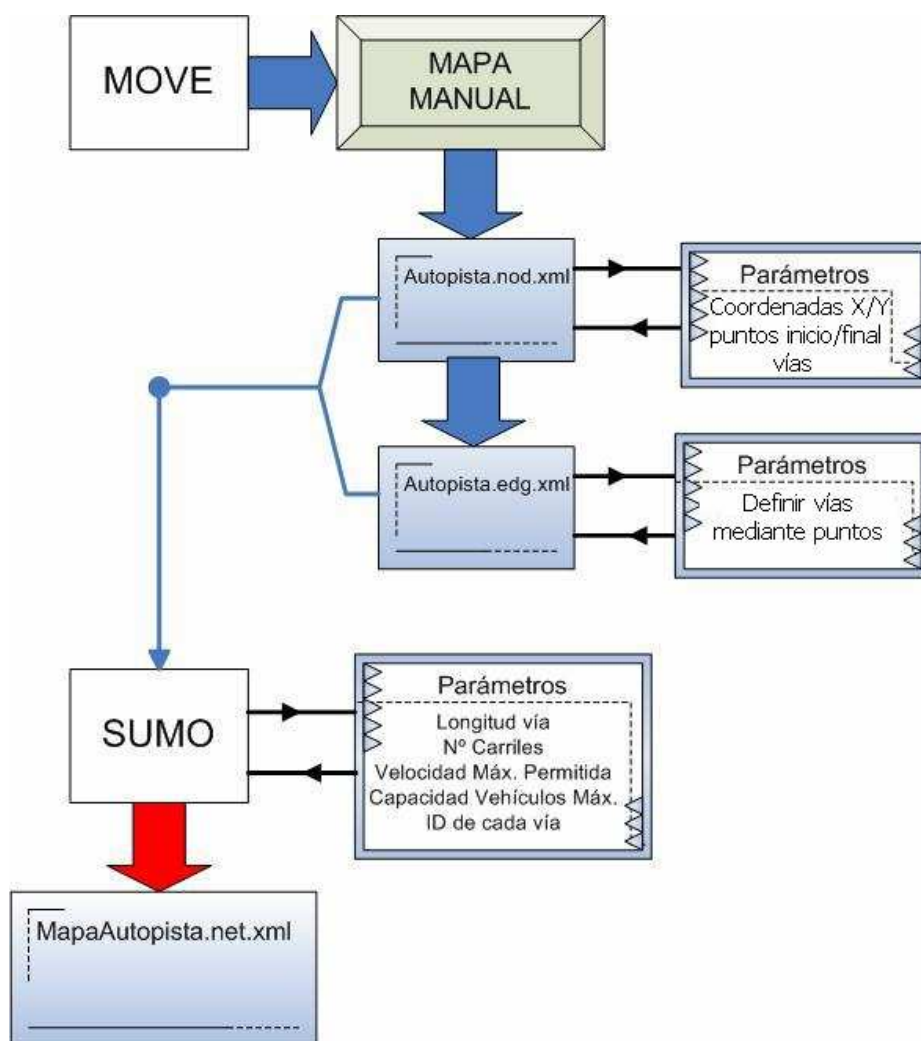
Figura B.1 Procedimiento para generar el mapa de la autopista
