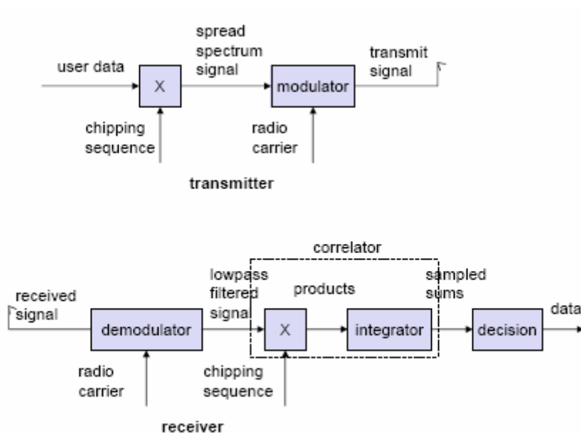
Figura 5.10 Esquema de modulación/demodulación mediante DSSS
