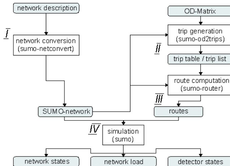
Figura 4.5 Proceso de simulación de SUMO, en gris los datos usados y en blanco las aplicaciones que intervienen
