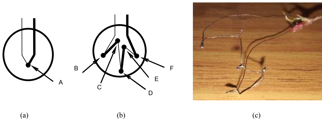
Figura 4. (a) conexión usual de una termocupla; (b) conexión en serie para sensar temperatura promedio; (c) fotografía de las del arreglo para sensar promedio y sus soldaduras.
