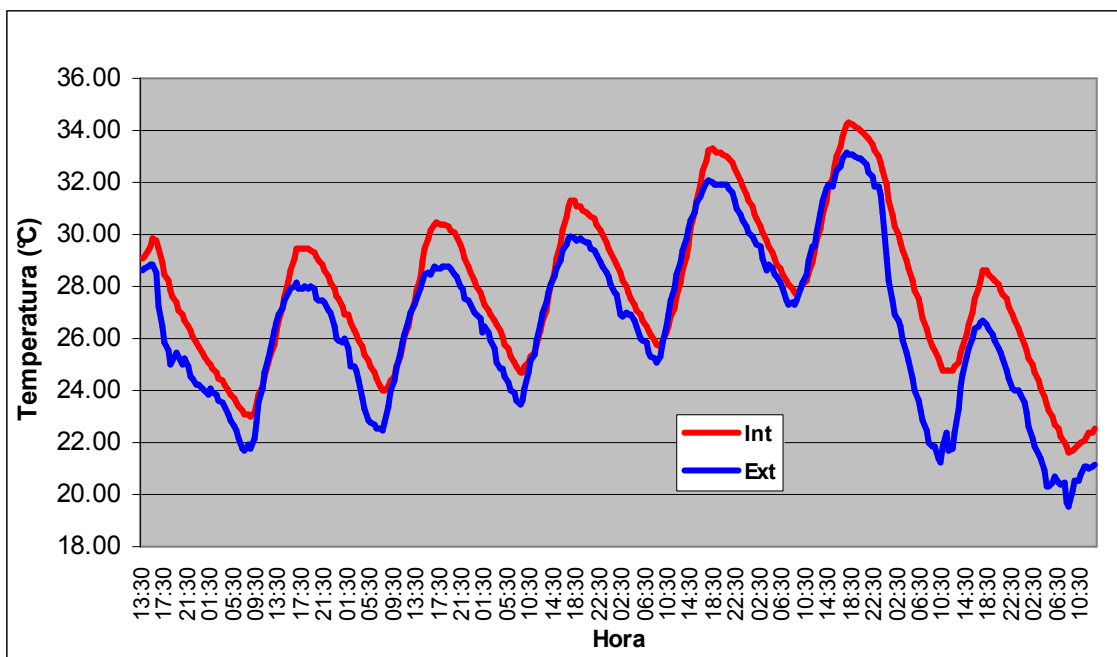
Fig. 9 y 10 –Balance de ganancias y pérdidas calculadas cada media hora entre las 13:30 hs del 24/01/2006 y las 12:30 hs del 31/01/2004 y su relación con las temperaturas interna y externa medidas.
