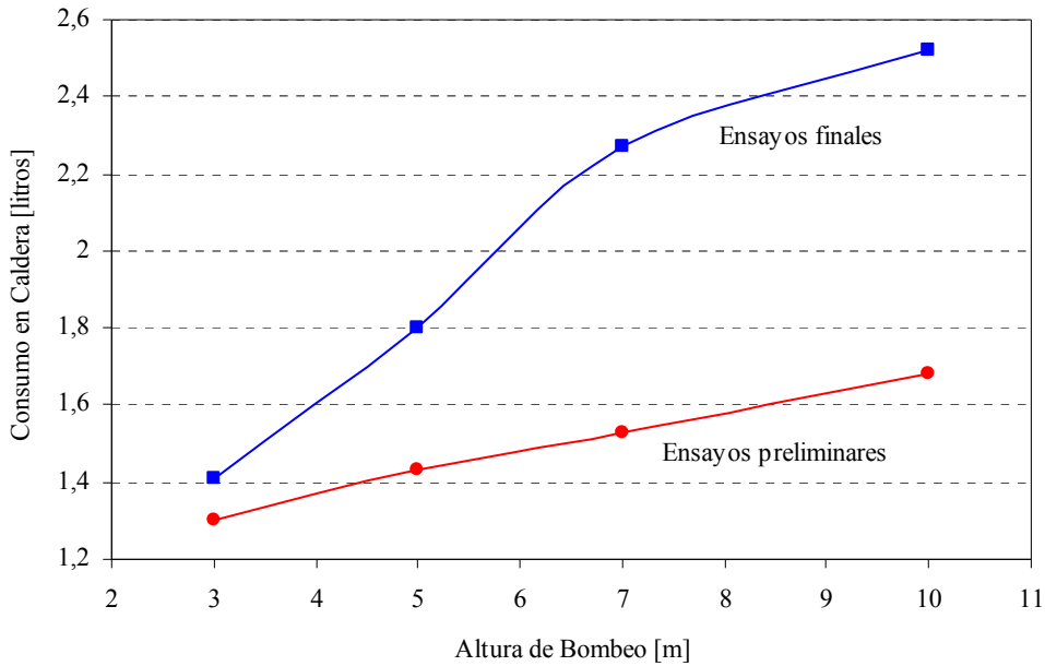
Fig.6. Variación del consumo de agua para diferentes presiones de carga
