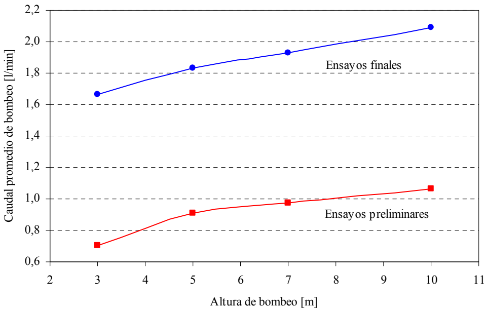
Fig. 7. Variación del caudal promedio de bombeo en función de la altura de bombeo
