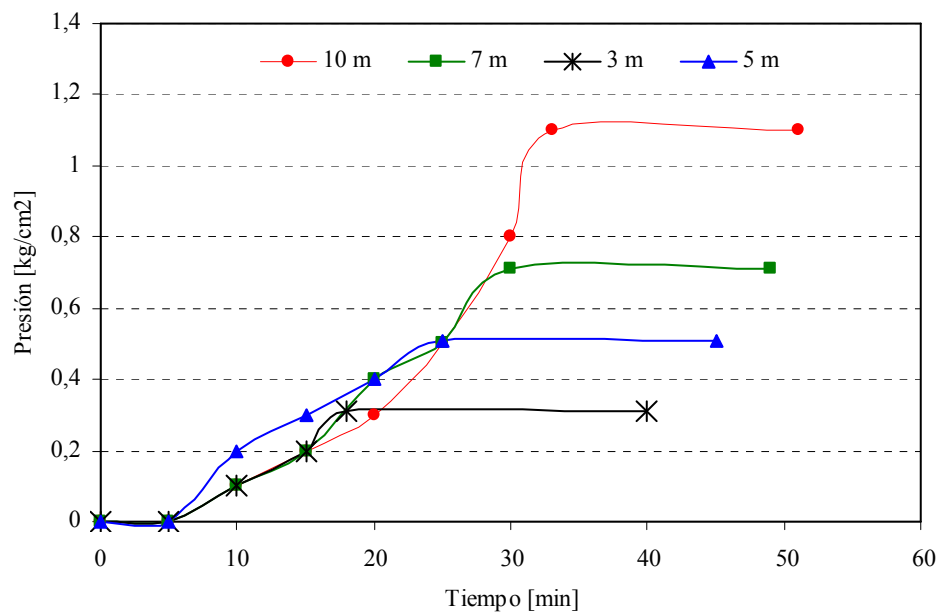
Fig. 5. Variación de la presión en la caldera en función del tiempo para distintas presiones de carga en el nuevo sistema.
