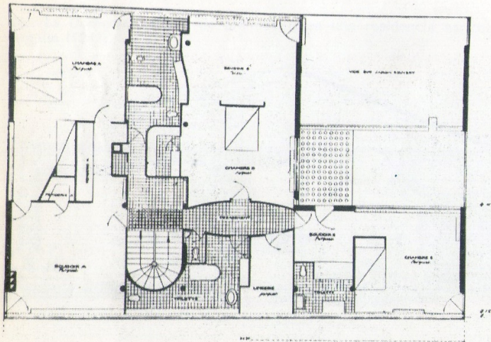
77. Le Corbusier, planta del segundo piso de chalet en Garches
