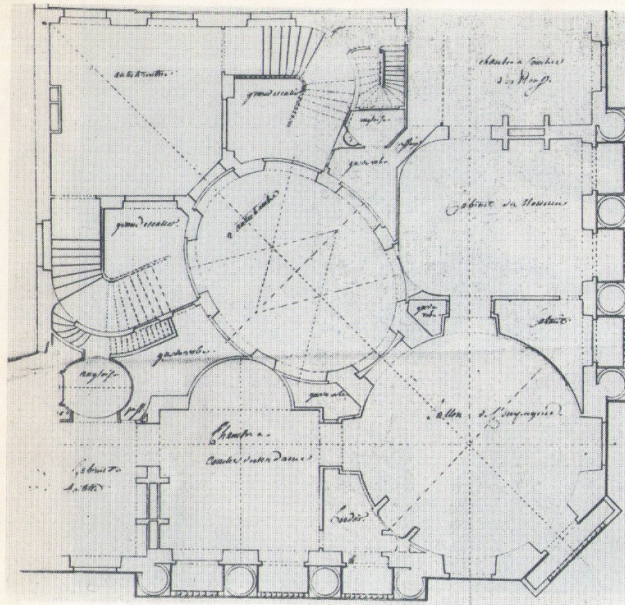
76. Ledoux, plano del Hotel de Montmorency, París (1770)
