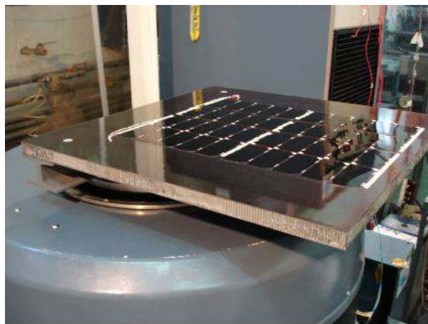
Figura 4. Montaje del panel en la base vibratoria para el ensayo de vibración cantilever .
