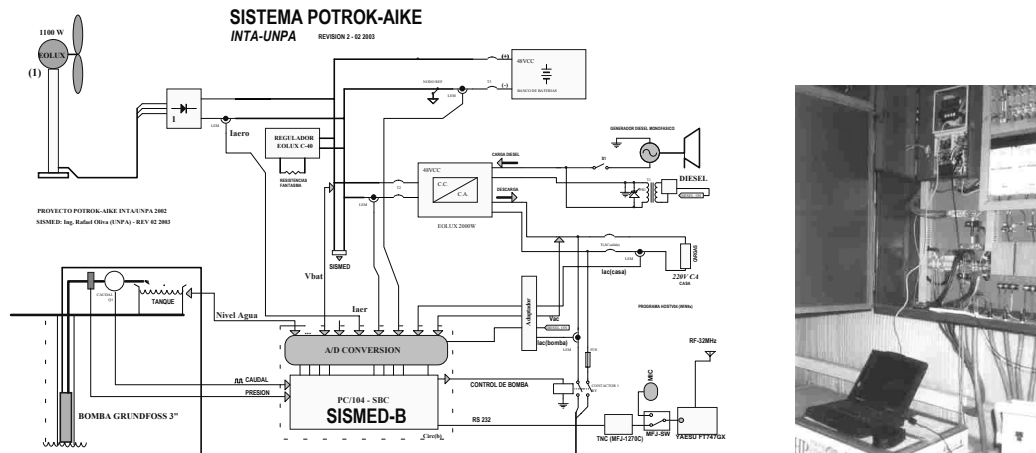
Figura 3a Diseño del Sistema para Potrok Aike. SISMED-B con Packet-Radio 3b (der.) Descarga SISMED01 E. Las Vegas
